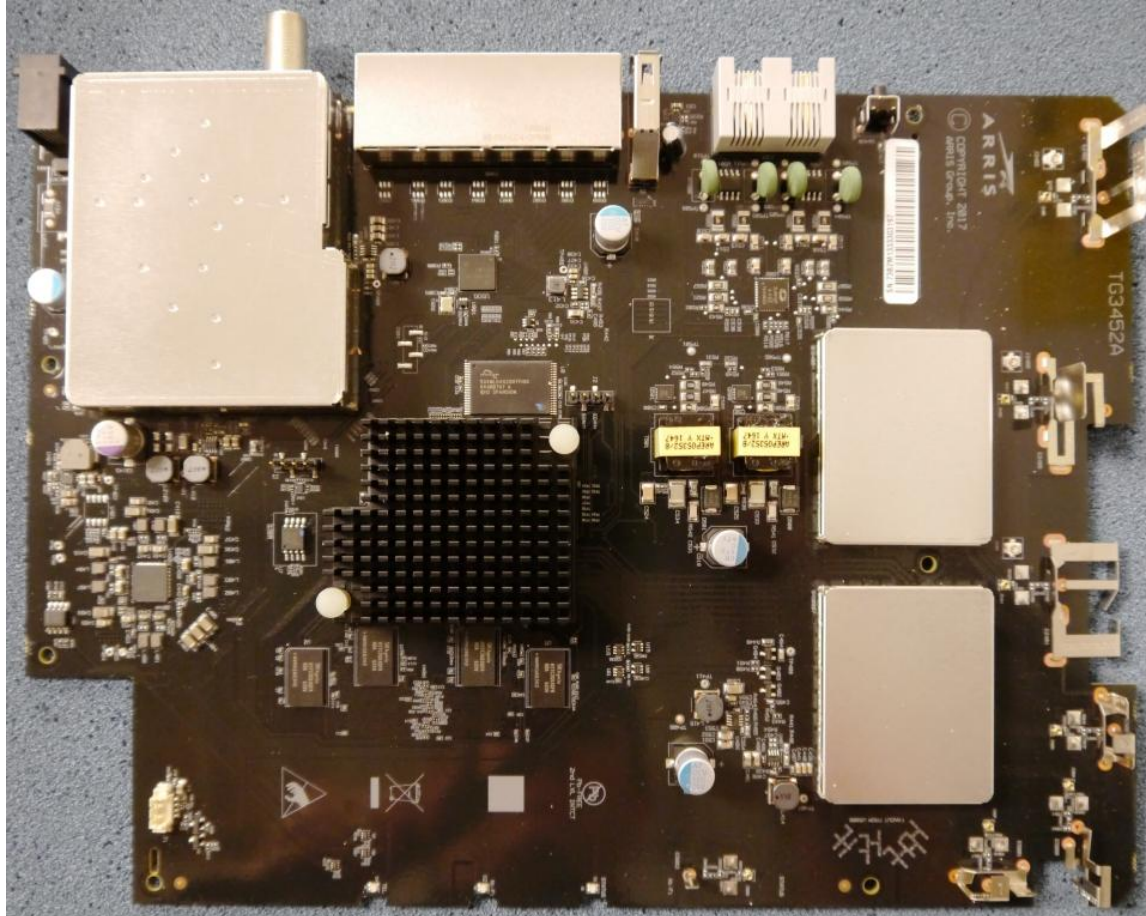
PCB - Top
