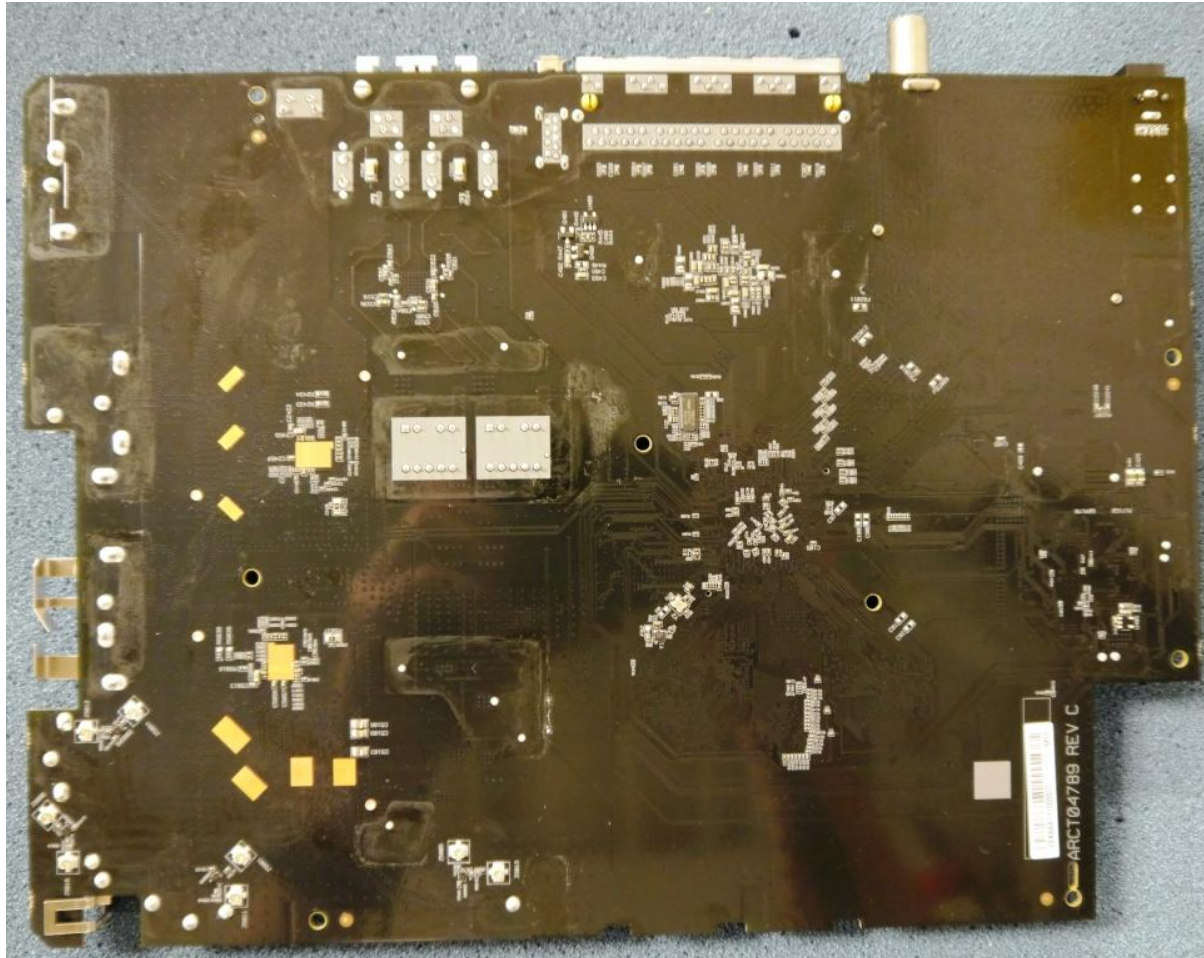
PCB Bottom
