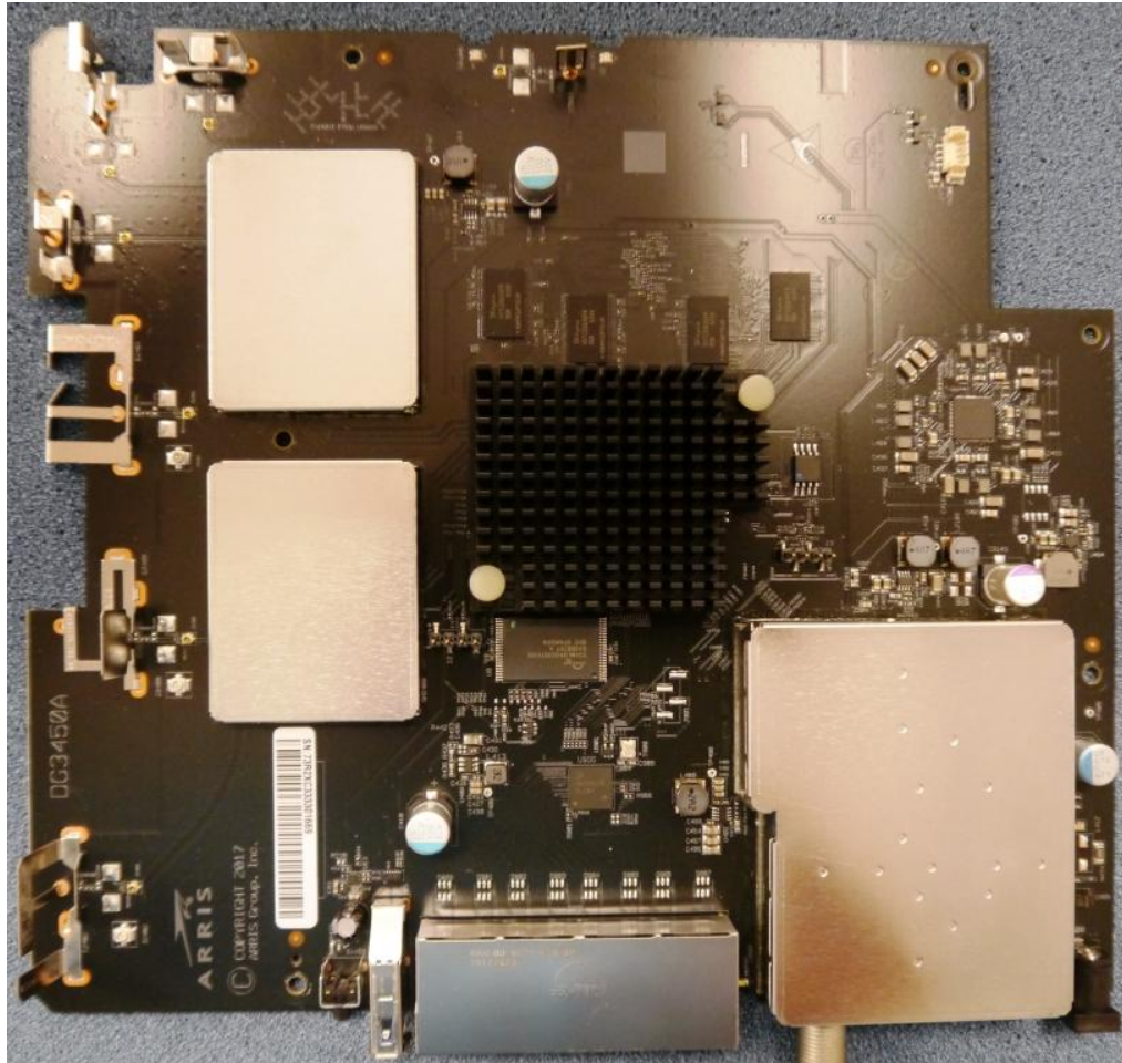
PCB - Top
