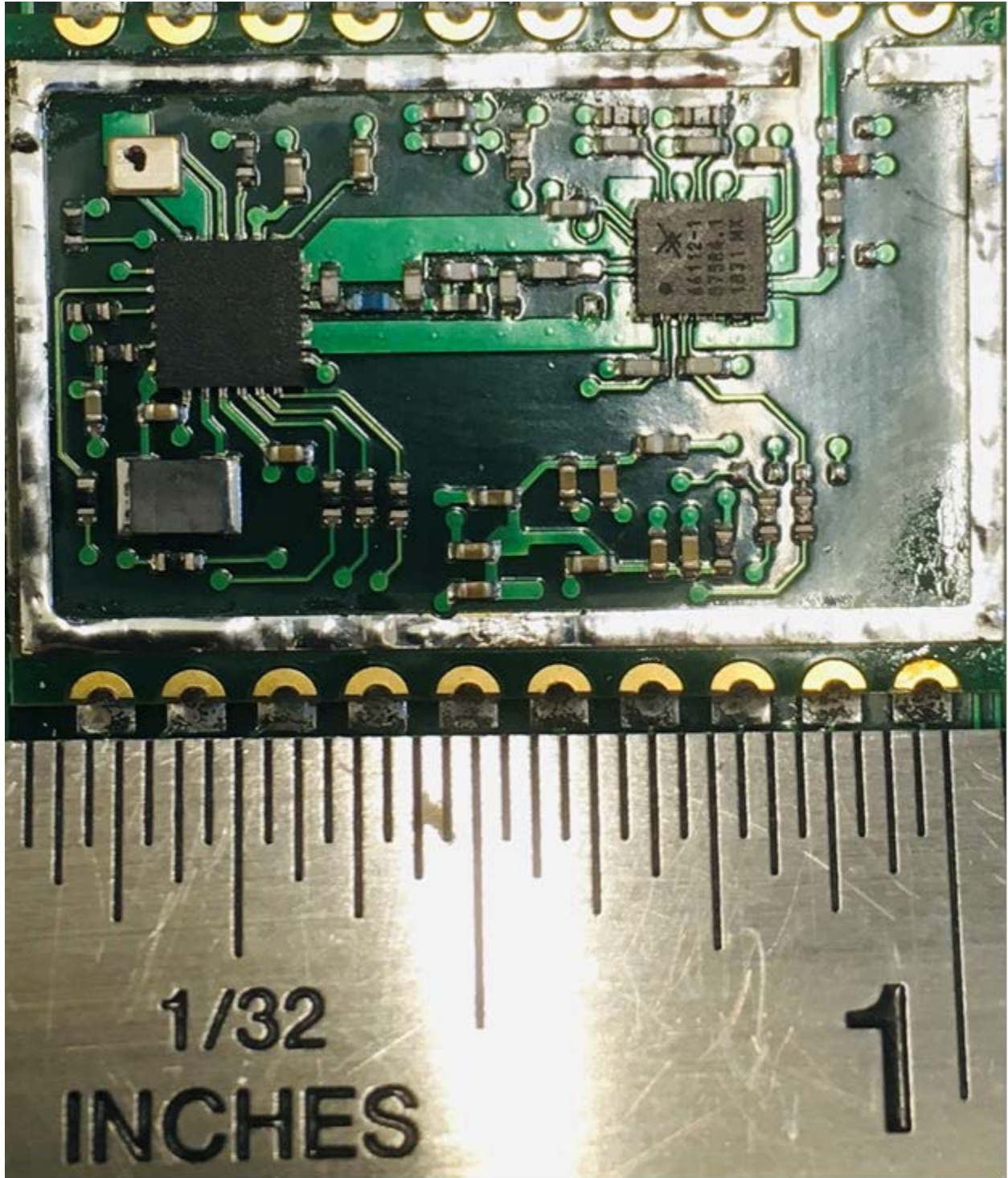
SX243 Module Internal Photos
