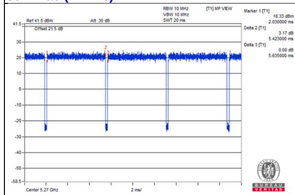
802.11ac (VHT40)
