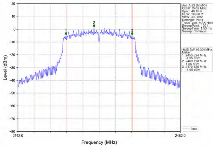
802.11n(HT20) HCH 2462MHz Ant2 (MIMO) NTNv
