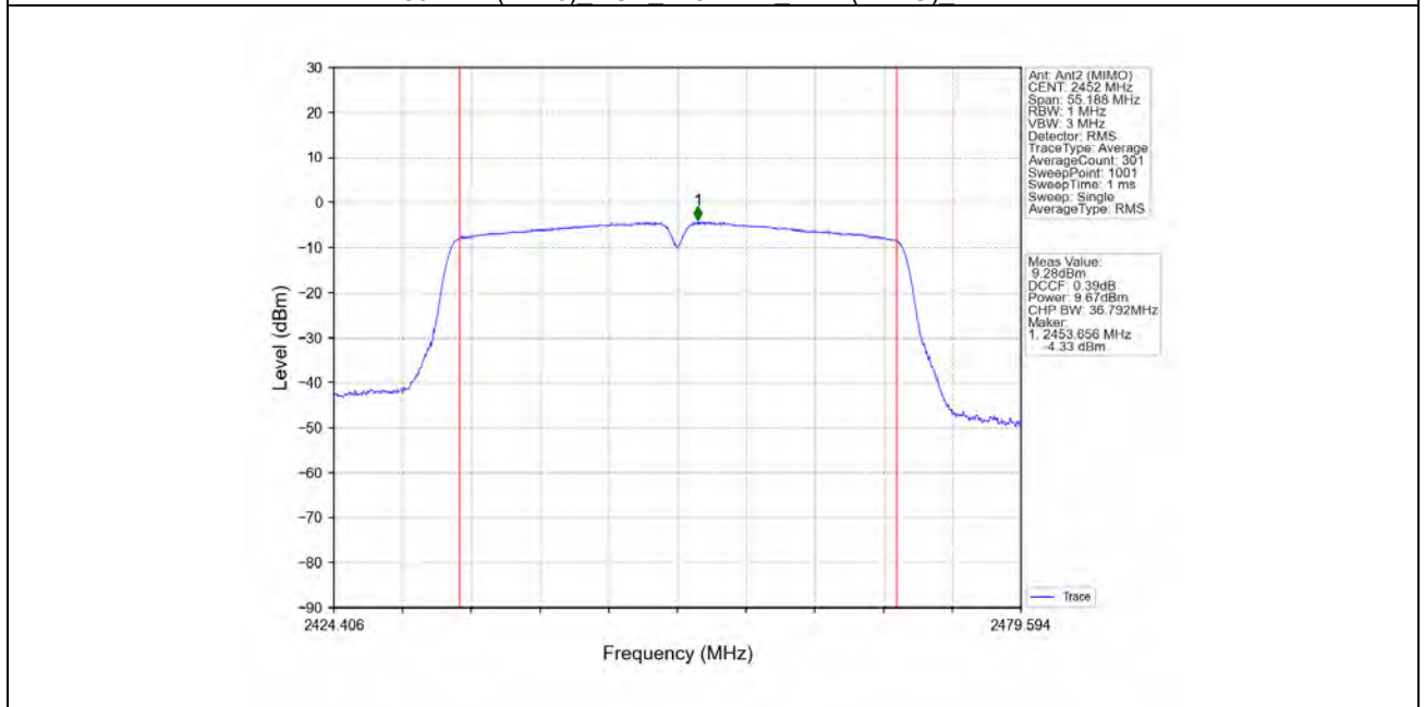
802.11n(HT40) HCH 2452MHz Ant2 (MIMO) NTNv
