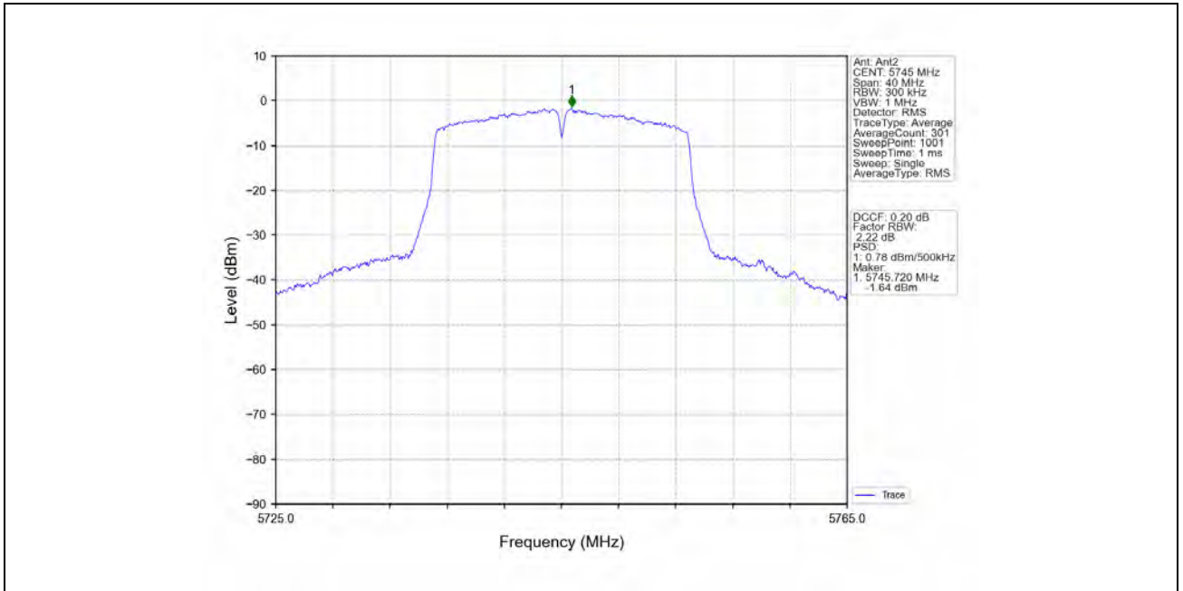
802.11ac(VHT20) LCH 5745MHz MIMO NTN
