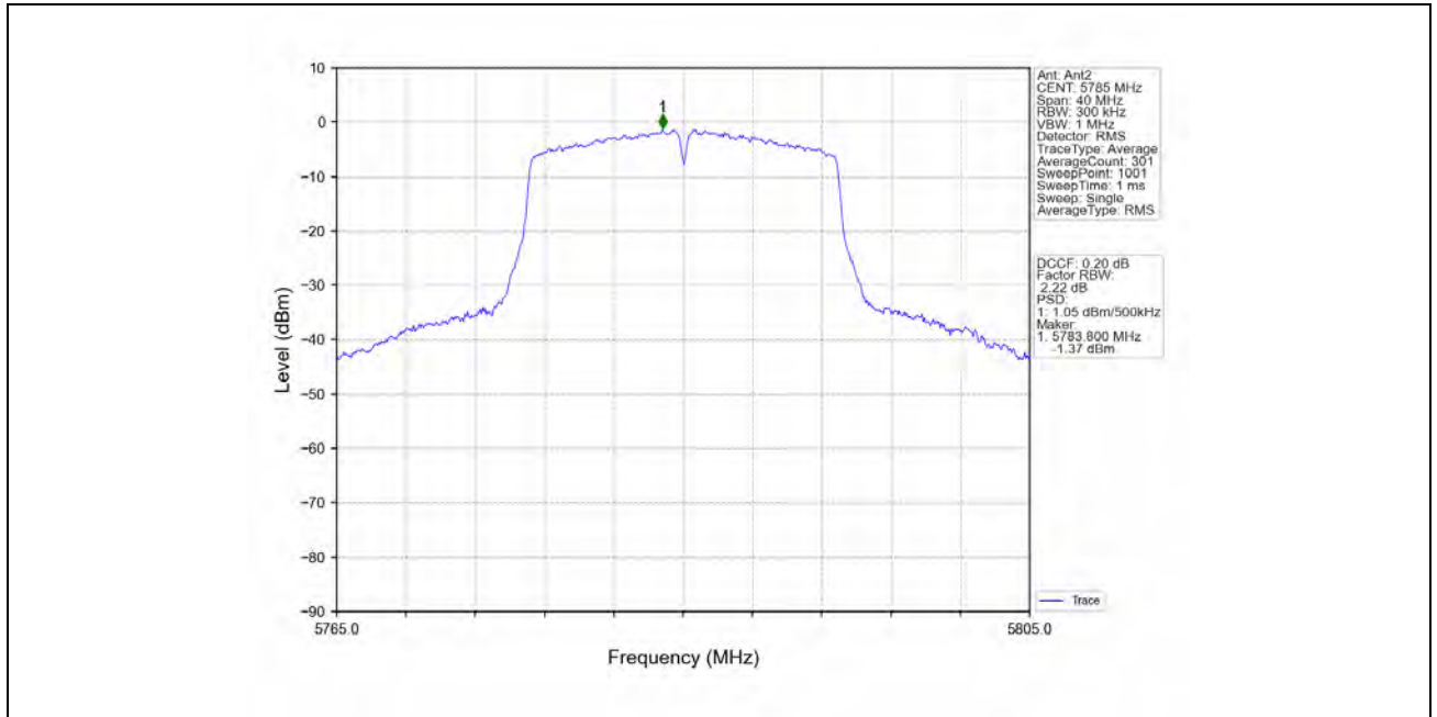
802.11n(HT20) MCH 5785MHz MIMO NTNv
