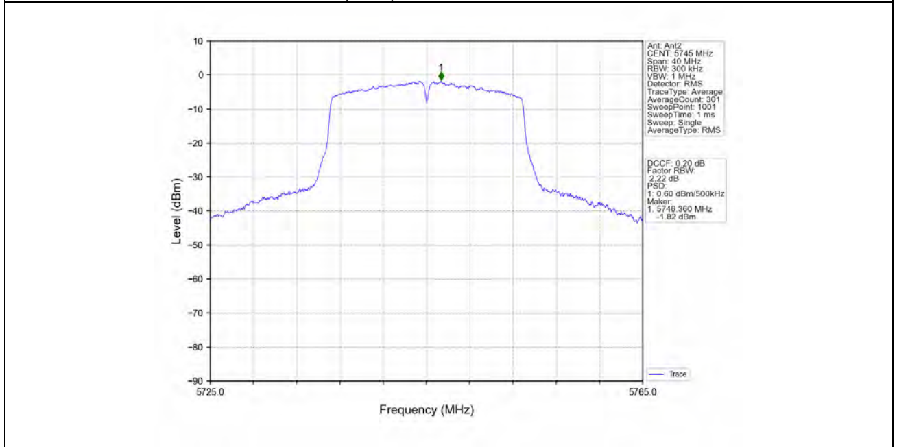
802.11n(HT20) LCH 5745MHz MIMO NTNv
