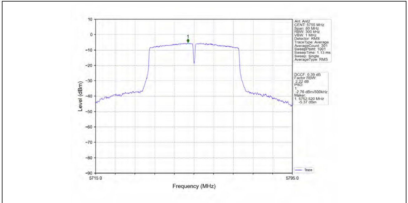
802.11n(HT40) LCH 5755MHz MIMO NTNv
