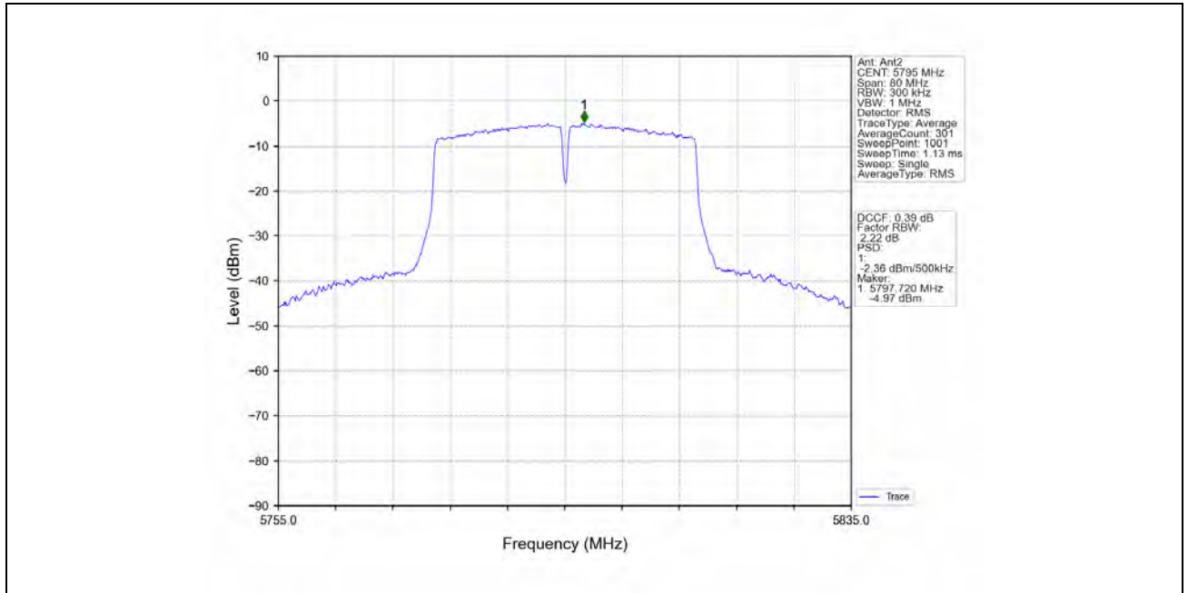
802.11ac(VHT40) HCH 5795MHz MIMO NTV
