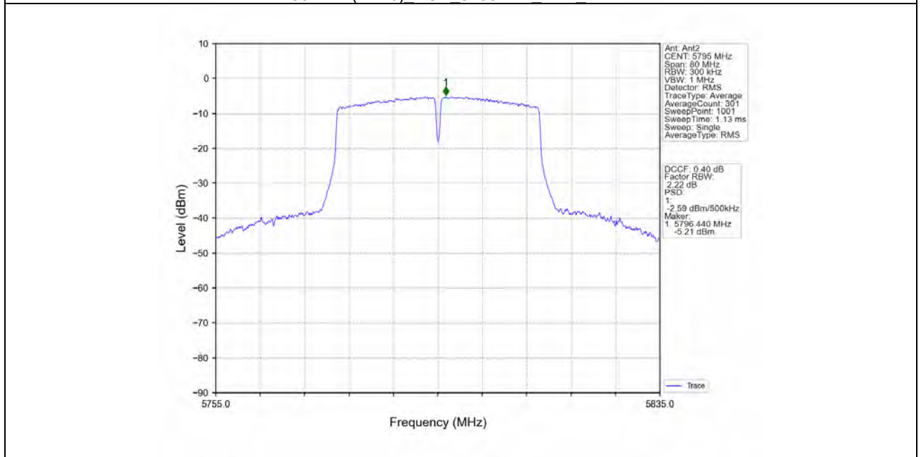
802.11n(HT40) HCH 5795MHz MIMO NTN
