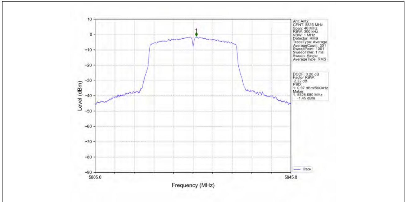
802.11ac(VHT20) HCH 5825MHz MIMO NTV
