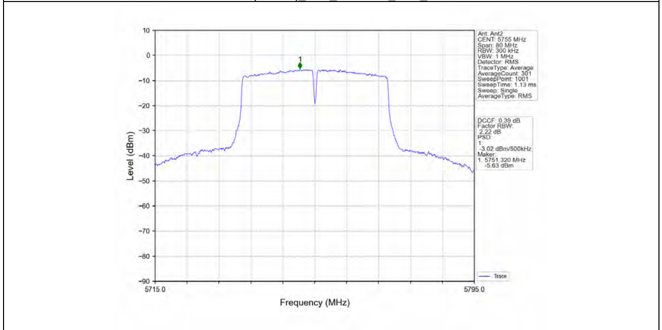
802.11ac(VHT40) LCH 5755MHz MIMO NTNv
