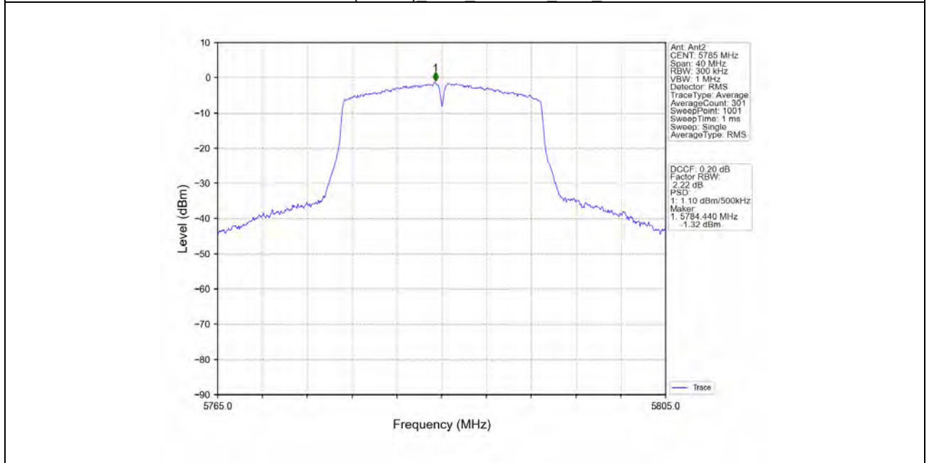
802.11ac(VHT20) MCH 5785MHz MIMO NTNv
