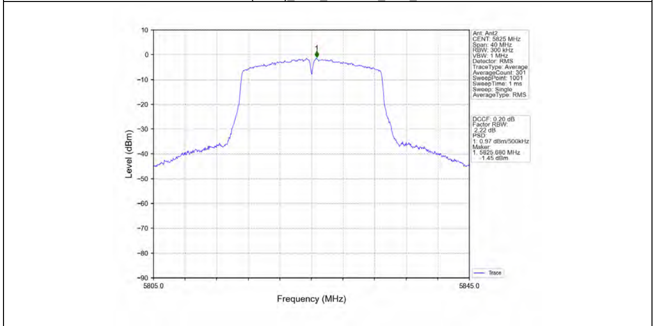
802.11n(HT20) HCH 5825MHz MIMO NTN
