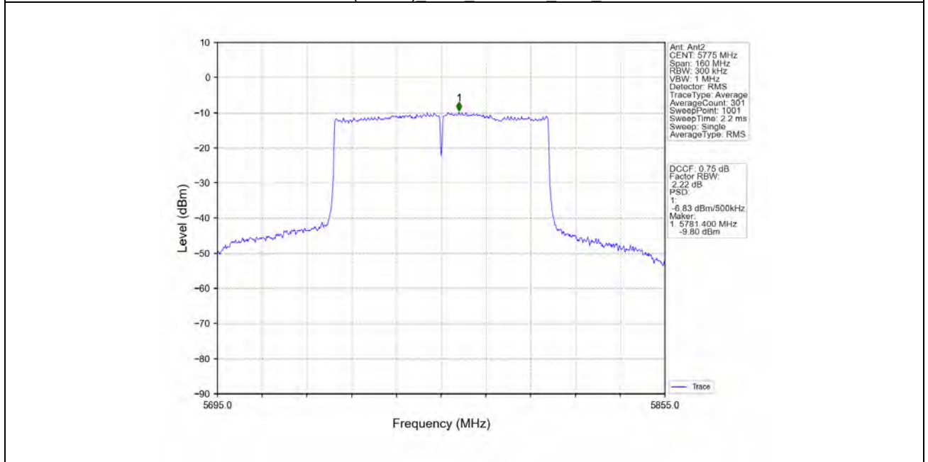
802.11ac(VHT80) MCH 5775MHz MIMO NTNv
