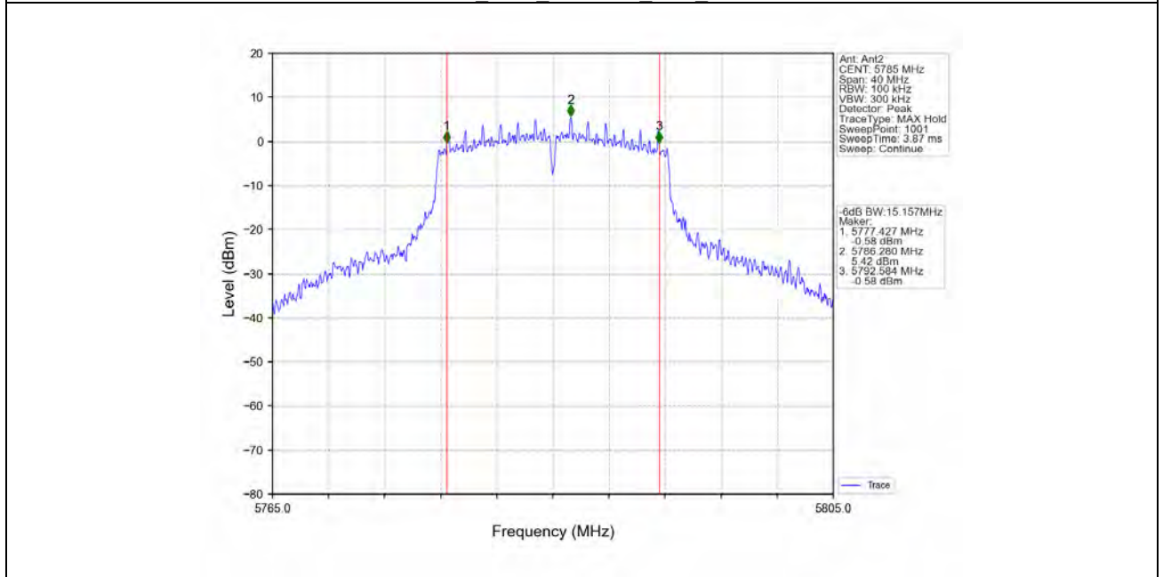
802.11a MCH 5785MHz Ant2 NTN
