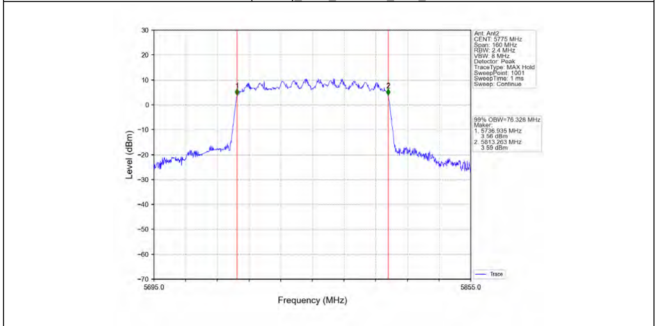
802.11ac(VHT80) MCH 5775MHz Ant2 NTN
