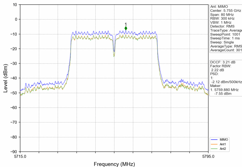
802.11n(HT40)_LCH_5755MHz_MIMO_NTNV
