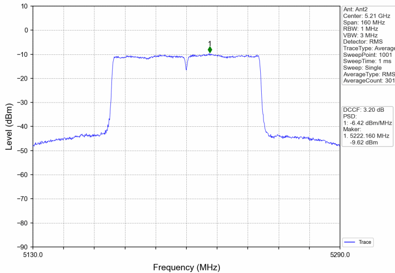
802.11ac(VHT80)_MCH_5210MHz_Ant2_NTNV
