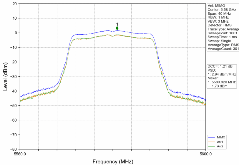
802.11n(HT20)_MCH_5580MHz_MIMO_NTNV
