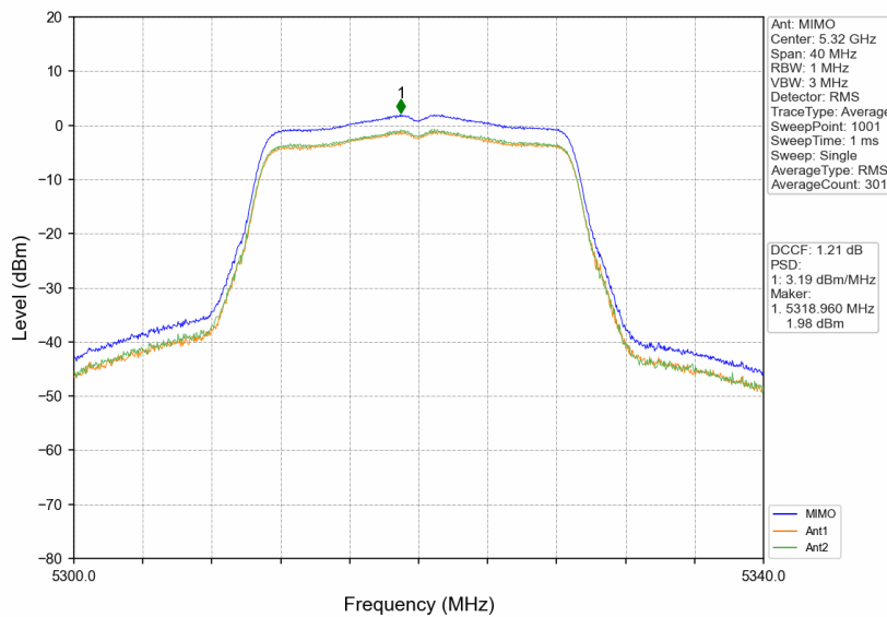
802.11n(HT20)_HCH_5320MHz_MIMO_NTNV
