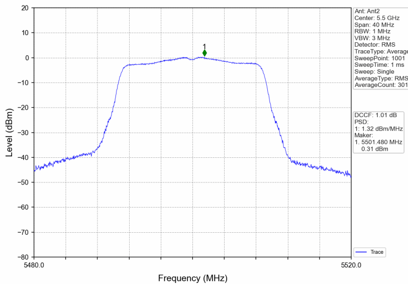
802.11n(HT20)_LCH_5500MHz_Ant2_NTNV
