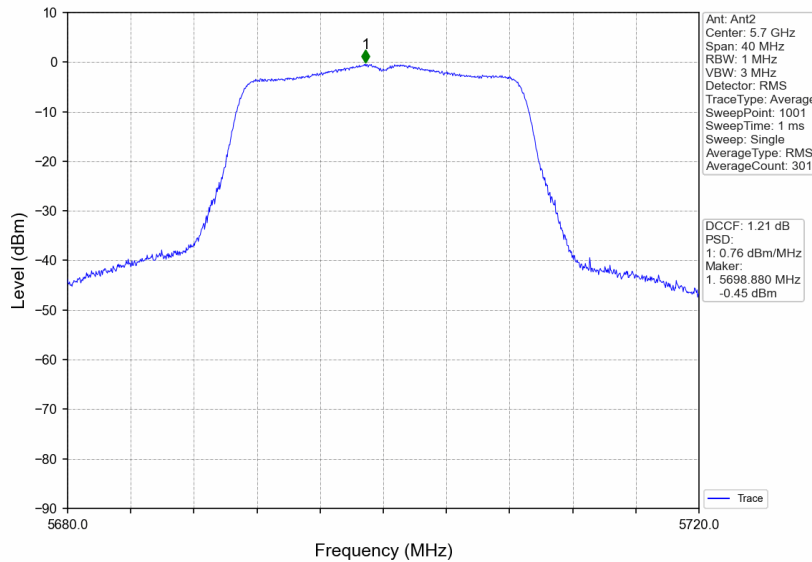
802.11n(HT20)_HCH_5700MHz_Ant2_NTNV
