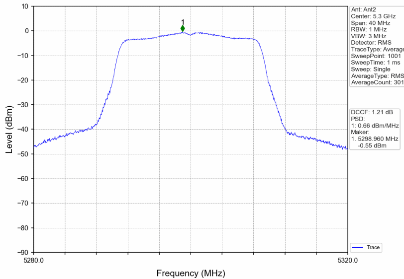
802.11n(HT20)_MCH_5300MHz_Ant2_NTNV
