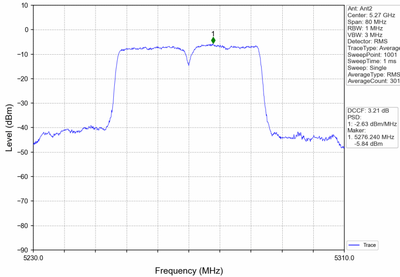
802.11n(HT40)_LCH_5270MHz_MIMO_NTNV
