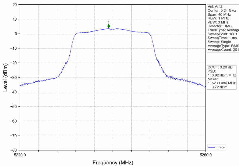
802.11a_HCH_5240MHz_Ant2_NTNV
