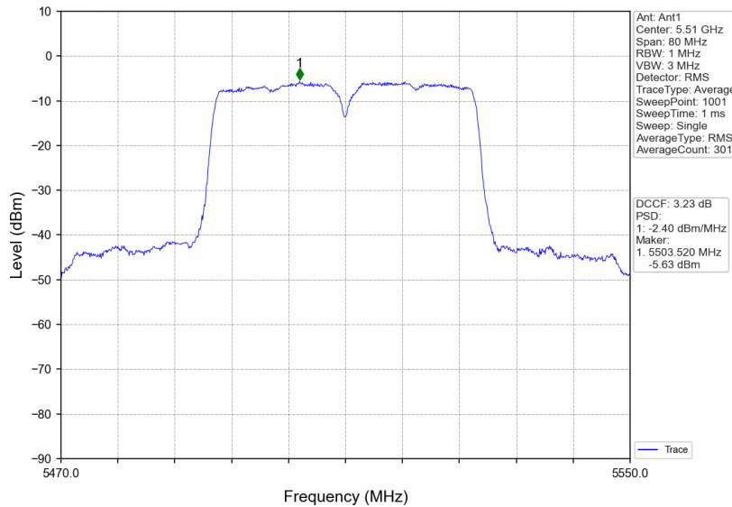
802.11n(HT40)_LCH_5510MHz_Ant1_NTNV
