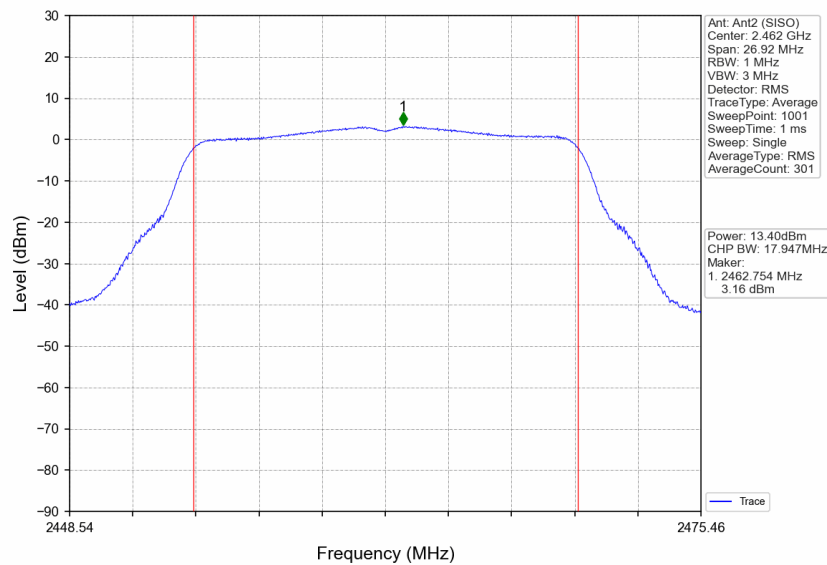
802.11g HCH 2462MHz Ant2 (SISO) NTVN
