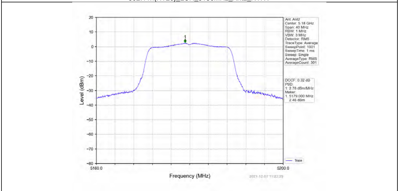
802.11n(HT20)_LCH_5180MHz_MIMO_NTNV
