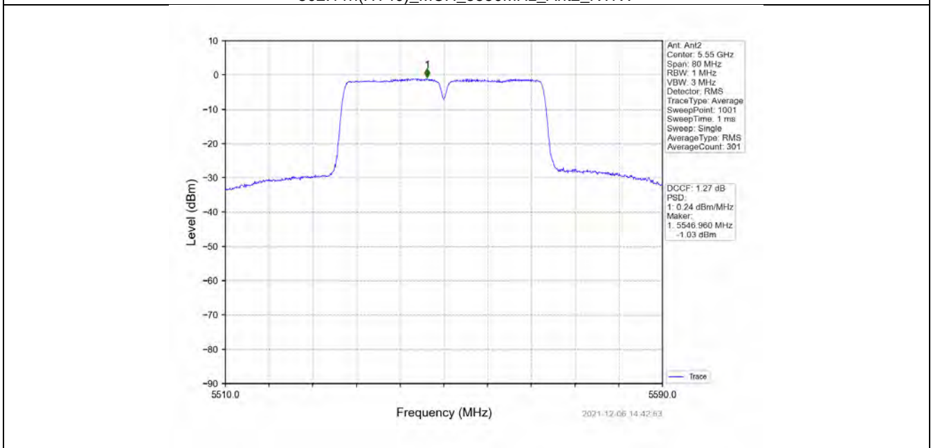
802.11n(HT40)_MCH_5550MHz_MIMO_NTNV
