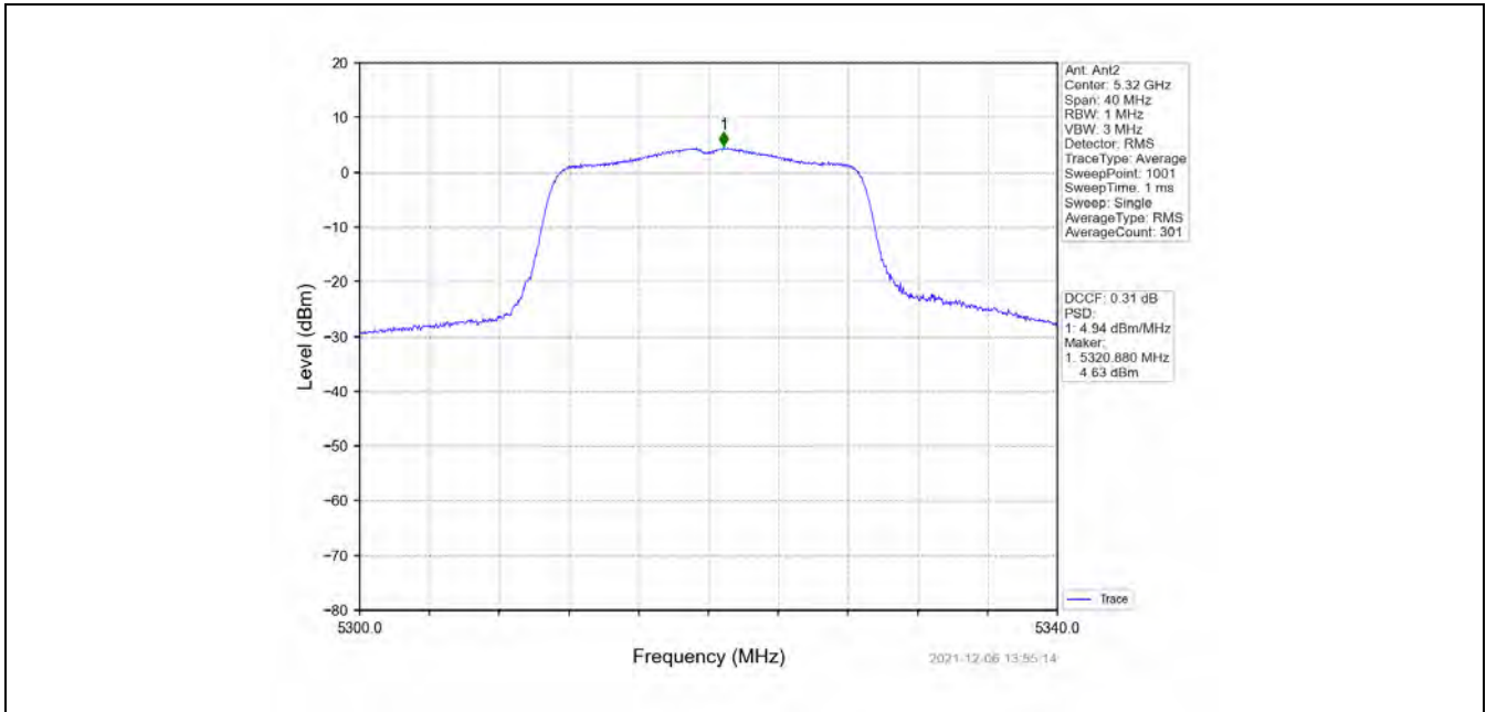
802.11n(HT20)_HCH_5320MHz_MIMO_NTNV
