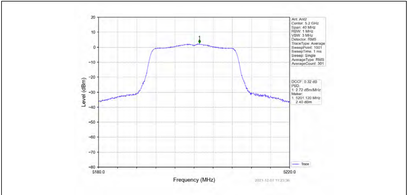
802.11n(HT20)_MCH_5200MHz_MIMO_NTNV
