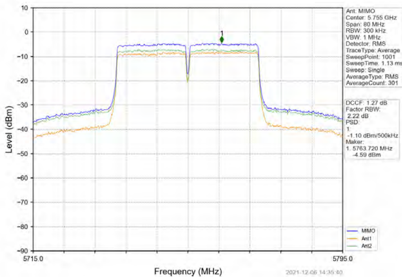
802.11n(HT40)_LCH_5755MHz_MIMO_NTNV
