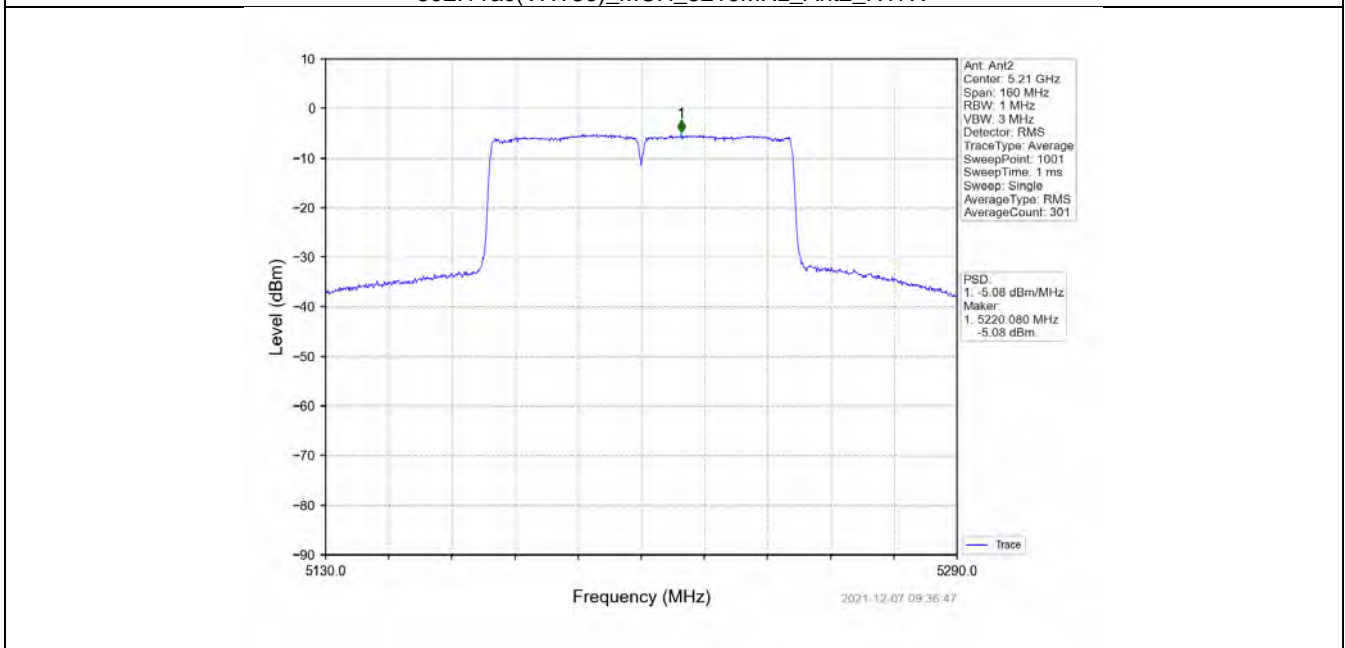
802.11ac(VHT80)_MCH_5210MHz_MIMO_NTNV
