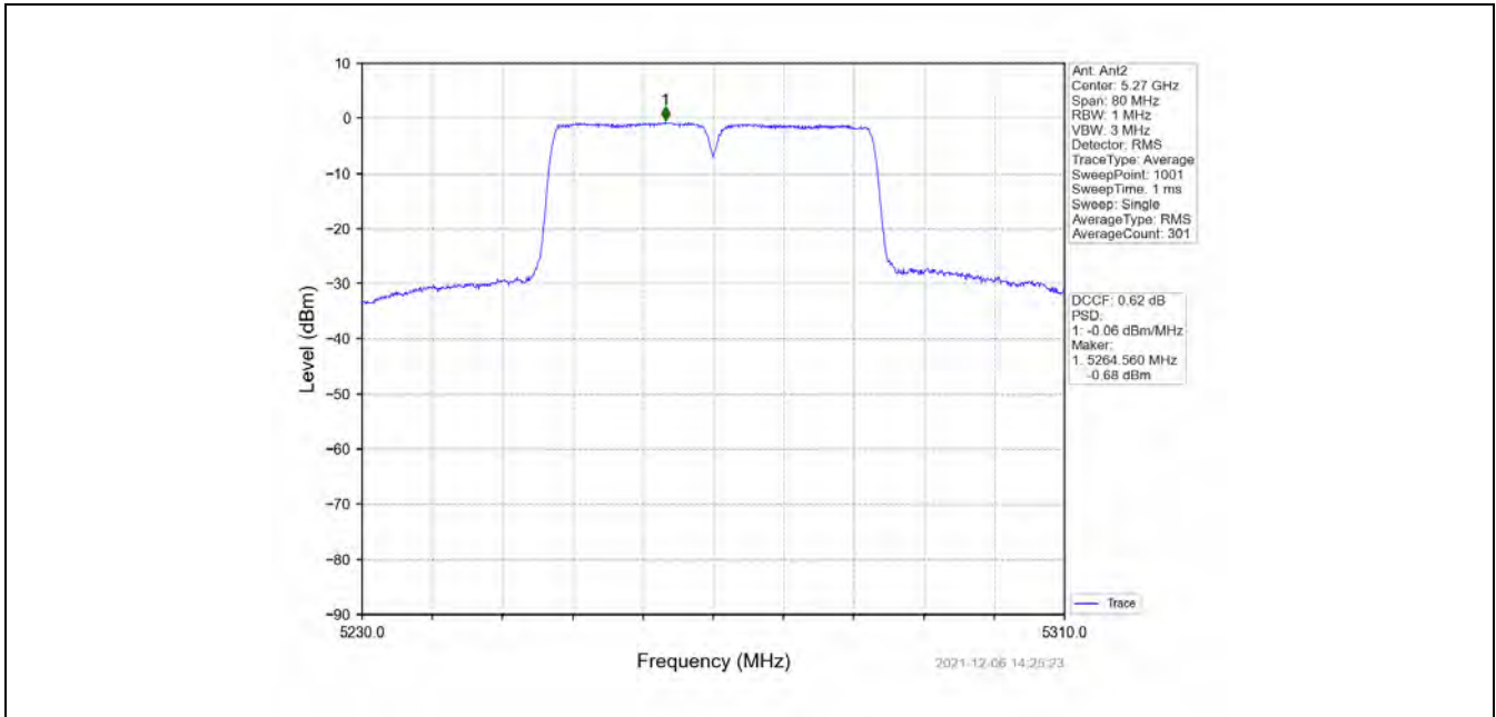
802.11n(HT40)_LCH_5270MHz_MIMO_NTNV
