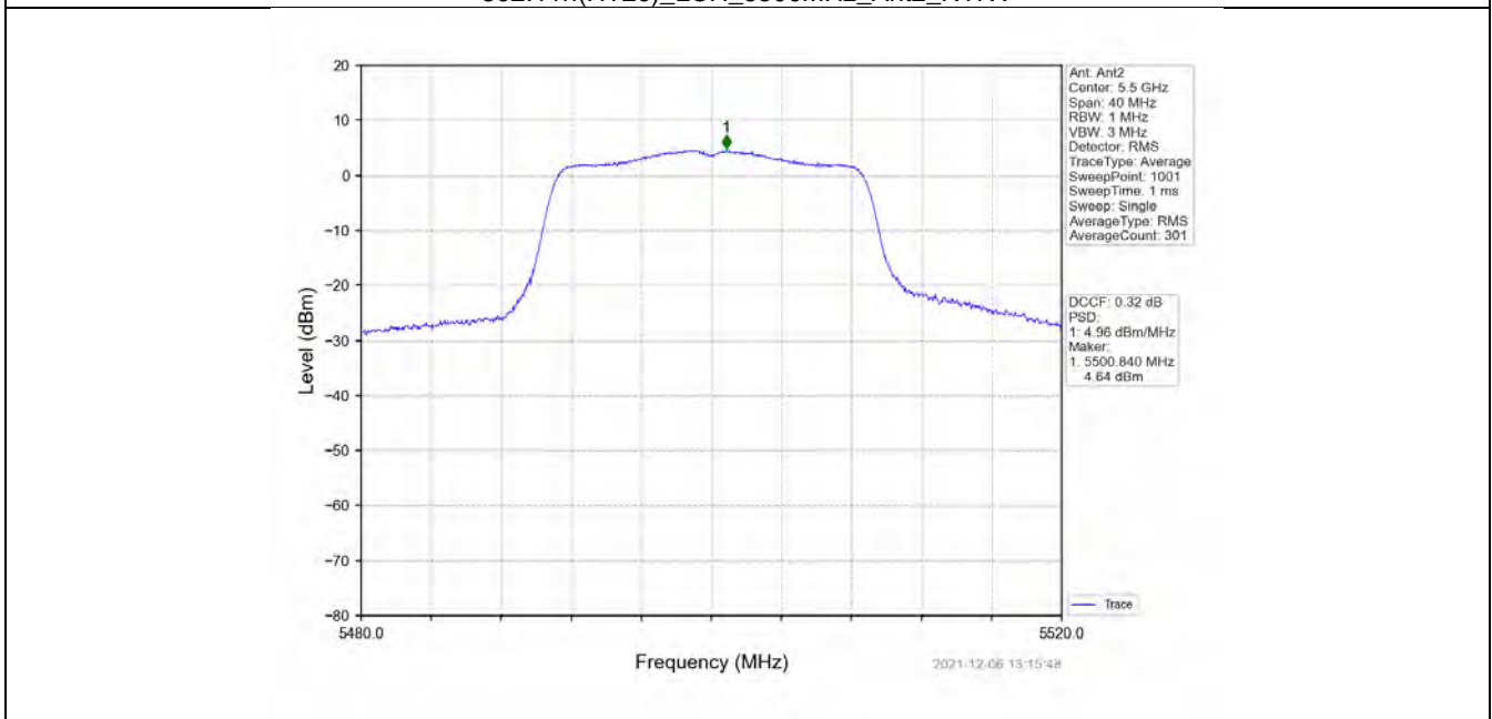
802.11n(HT20)_LCH_5500MHz_MIMO_NTNV
