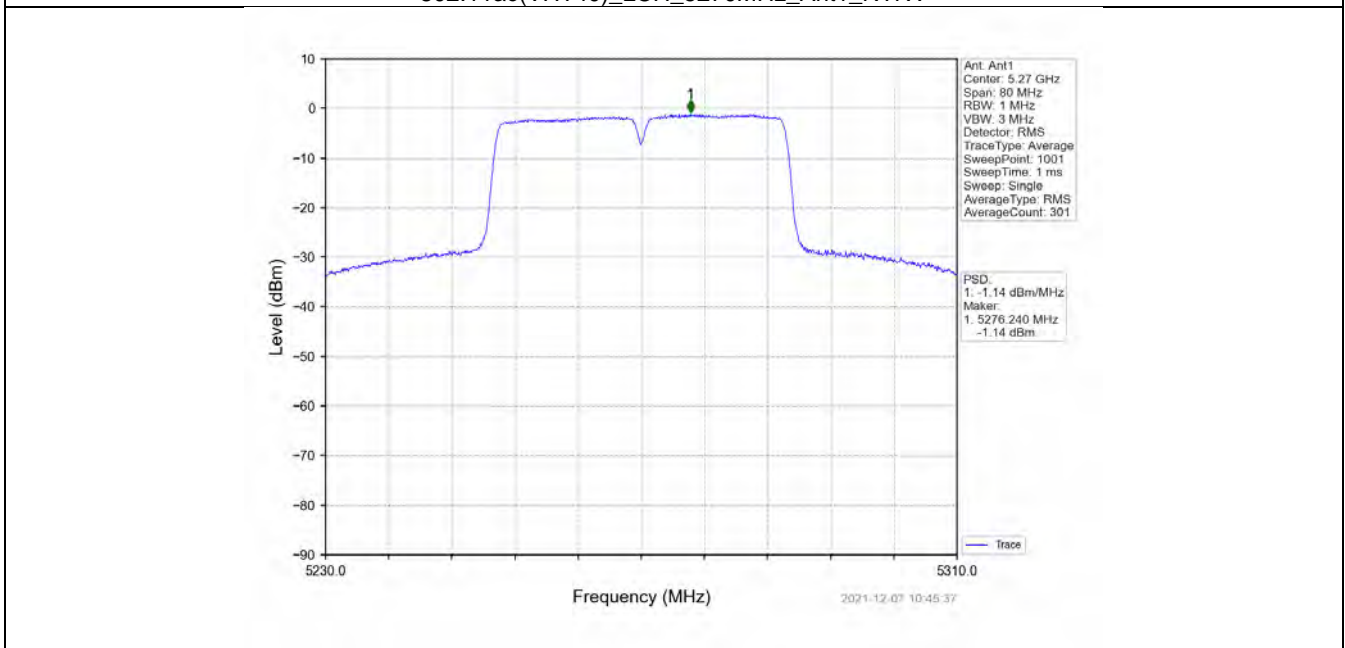
802.11ac(VHT40)_LCH_5270MHz_Ant2_NTNV
