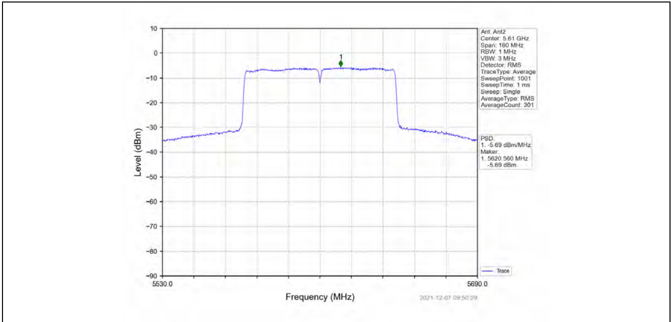
802.11ac(VHT80)_HCH_5610MHz_MIMO_NTNV
