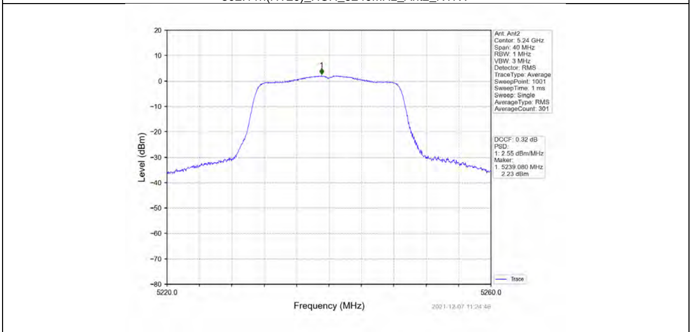
802.11n(HT20)_HCH_5240MHz_MIMO_NTNV
