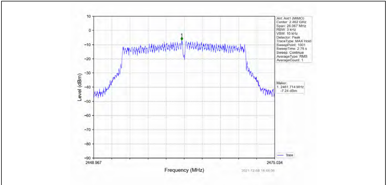
802.11n(HT20)_HCH_2462MHz_MIMO_NTNV
