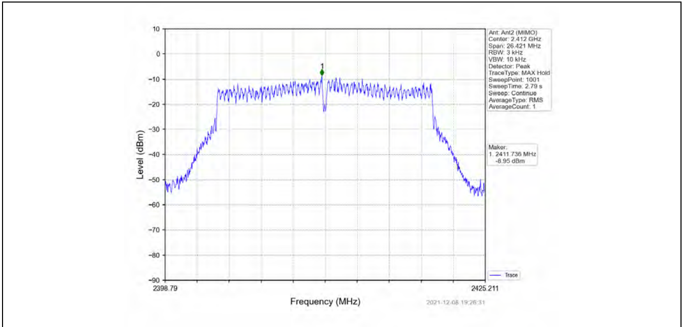
802.11n(HT20)_LCH_2412MHz_MIMO_NTNV
