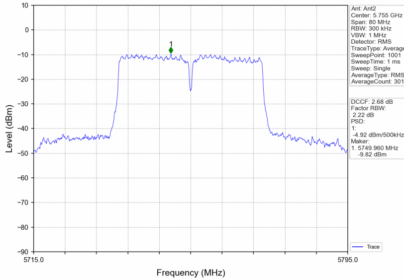
802.11n(HT40)_LCH_5755MHz_MIMO_NTNV
