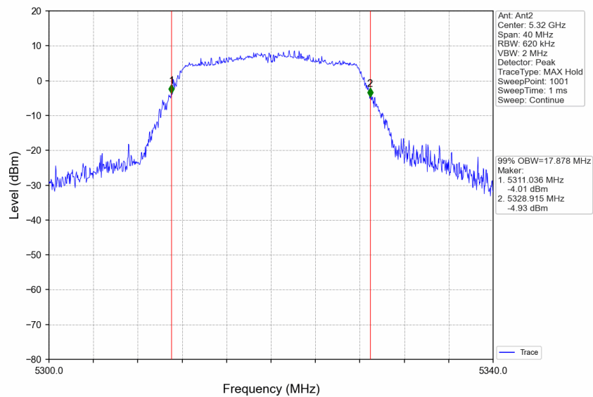
802.11a_HCH_5320MHz_Ant2_NTNV
