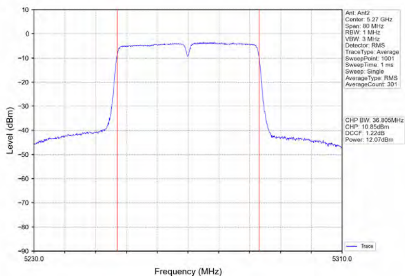
802.11ac(VHT40) LCH_5270MHz_Ant2_NTNV
