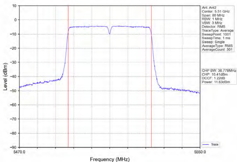
802.11ac(VHT40) LCH_5510MHz_Ant2_NTNV
