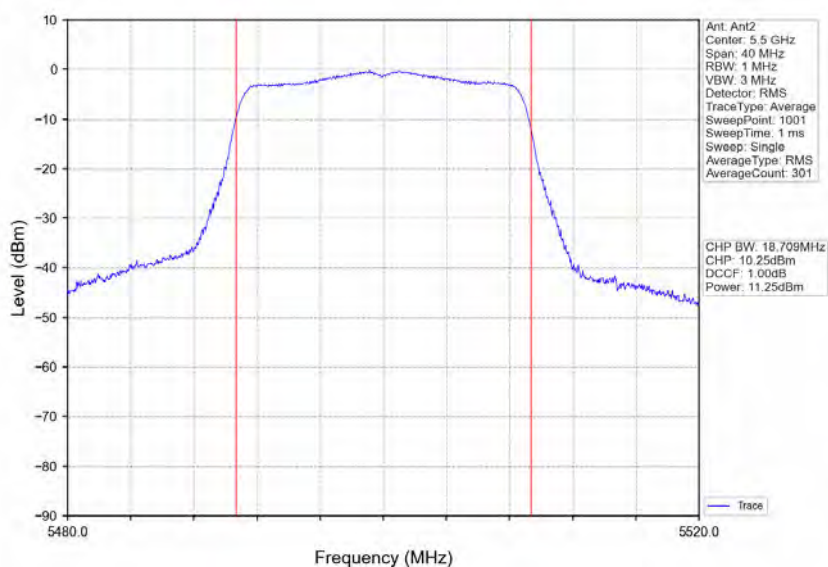
802.11ac(VHT20) LCH_5500MHz_Ant2_NTNV
