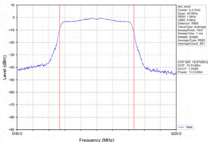
802.11n(HT20)_MCH_5200MHz_Ant2_NTNV
