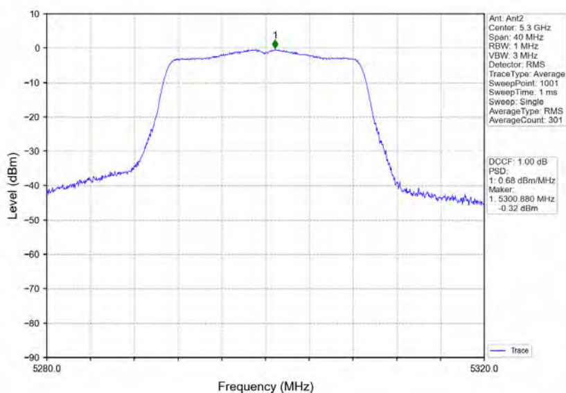
802.11n(HT20)_MCH_5300MHz_Ant2_NTNV
