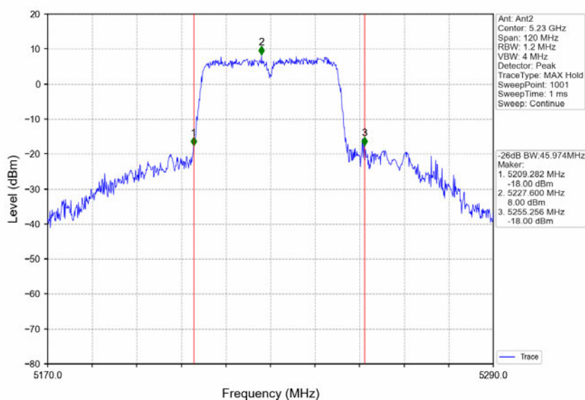
802.11n(HT40)_HCH_5230MHz_Ant2_NTNV
