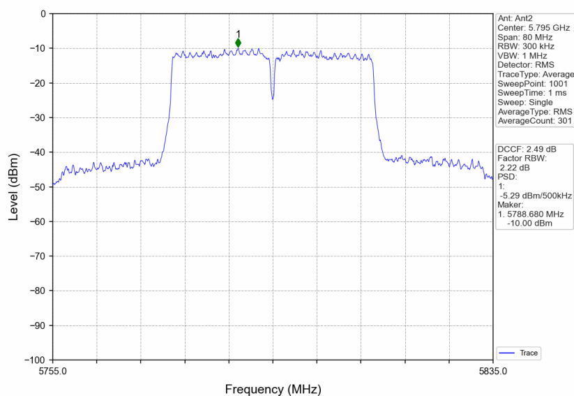
802.11n(HT40)_HCH_5795MHz_Ant2_NTNV
