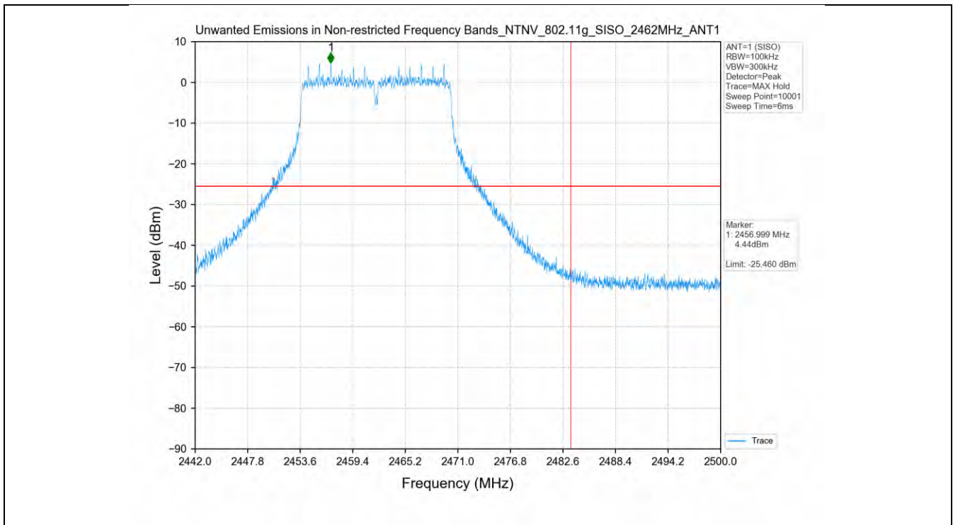
802.11g_2462MHz_SISO_ANT1
