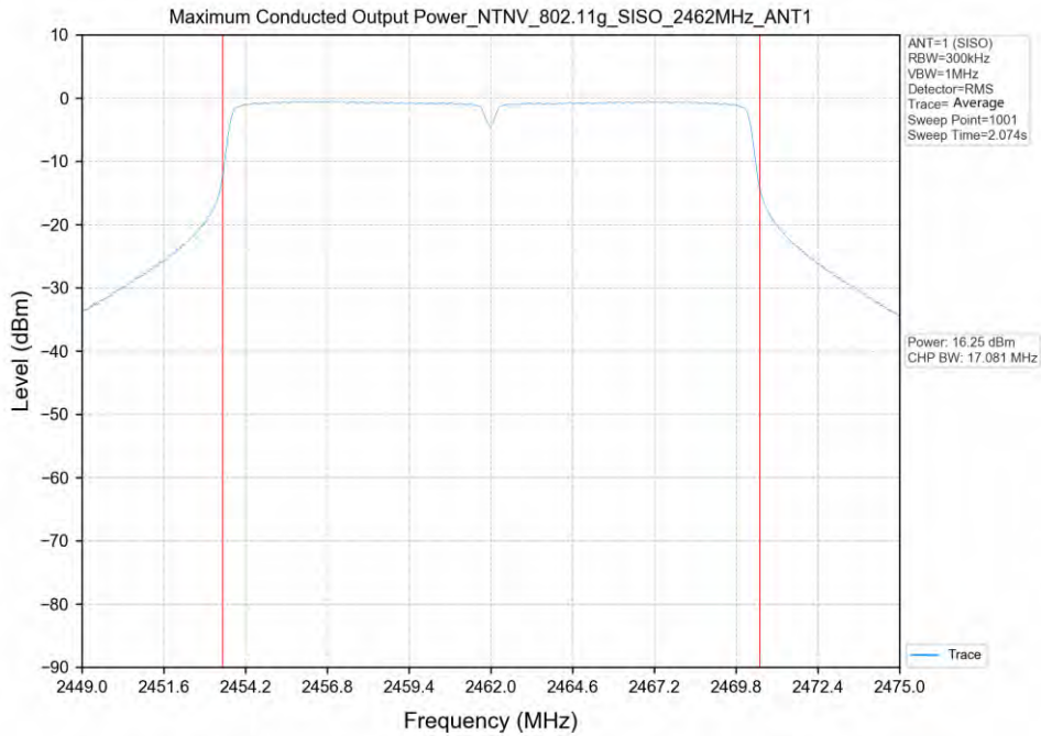
802.11g_2462MHz_SISO_ANT1
