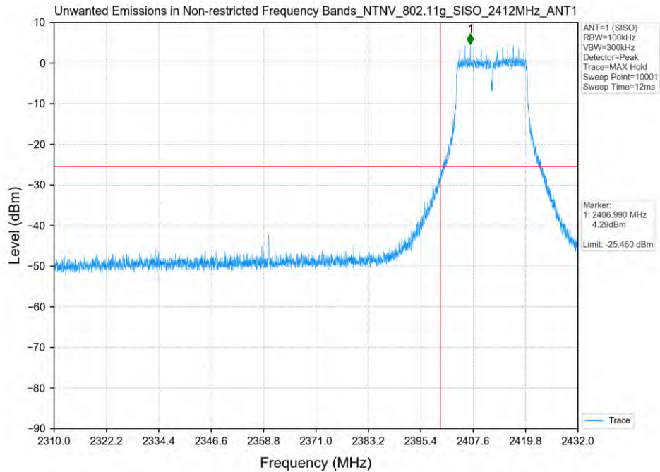
802.11g_2412MHz_SISO_ANT1
