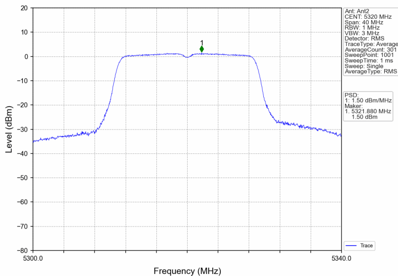
802.11n(HT20)_HCH_5320MHz_Ant2_NTNV
