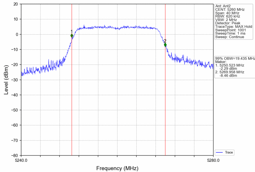
802.11n(HT20)_LCH_5260MHz_Ant2_NTNV
