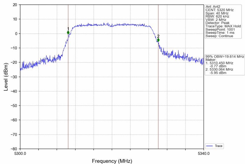
802.11n(HT20)_HCH_5320MHz_Ant2_NTNV
