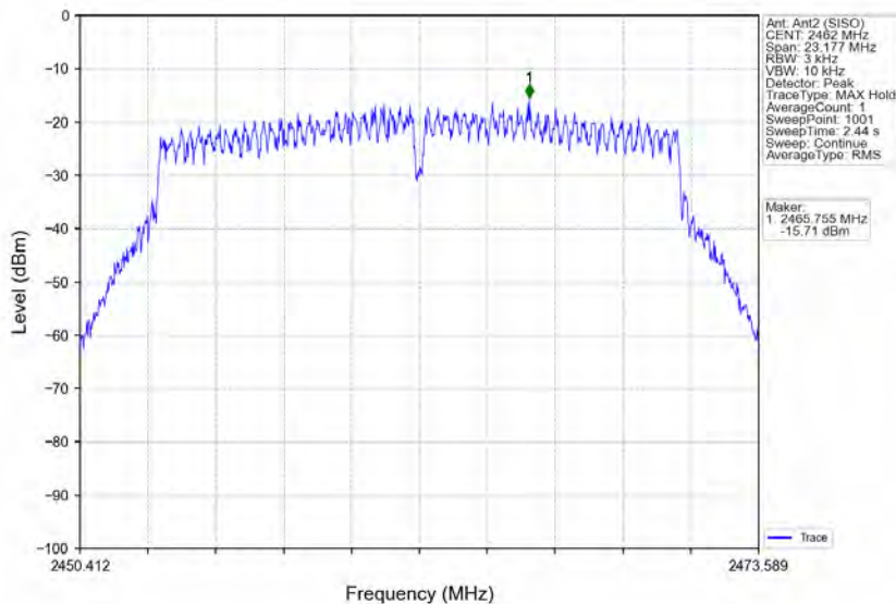
802.11n(HT20)_HCH_2462MHz_Ant2 (SISO)_NTNV
