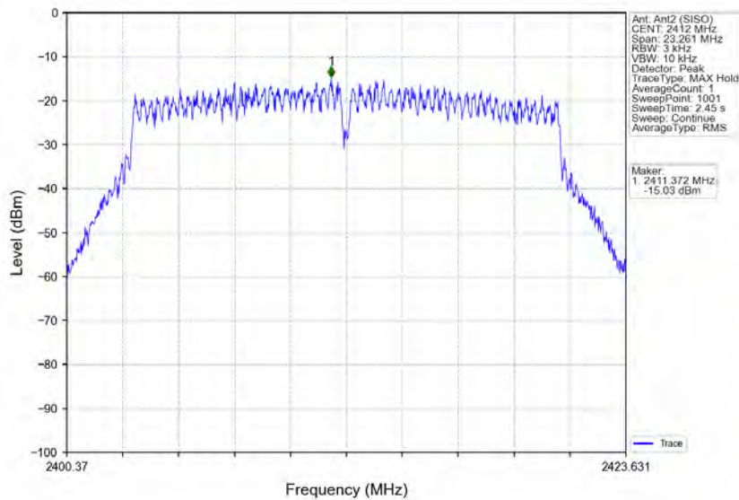
802.11n(HT20)_LCH_2412MHz_Ant2 (SISO)_NTNV
