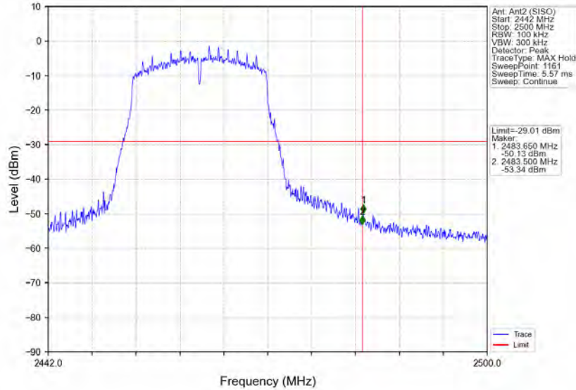
802.11n(HT20)_HCH_2462MHz_Ant2 (SISO)_NTNV
