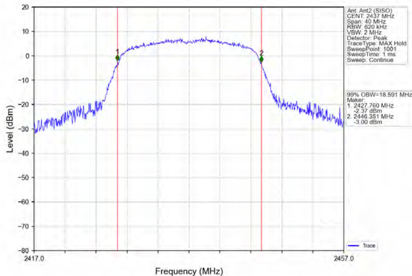
802.11n(HT20)_MCH_2437MHz_Ant2 (SISO)_NTNV
