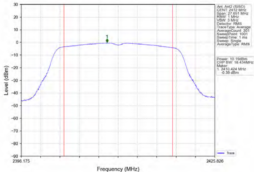
802.11n(HT20)_LCH_2412MHz_Ant2 (SISO)_NTNV
