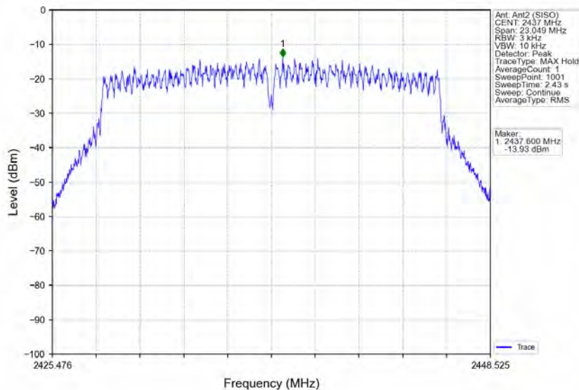
802.11n(HT20)_MCH_2437MHz_Ant2 (SISO)_NTNV
