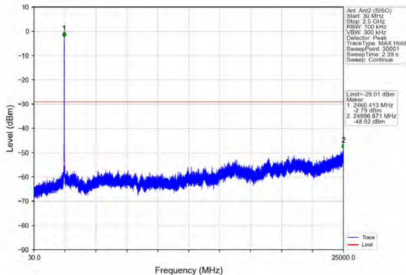
802.11n(HT20)_HCH_2462MHz_Ant2 (SISO)_NTNV
