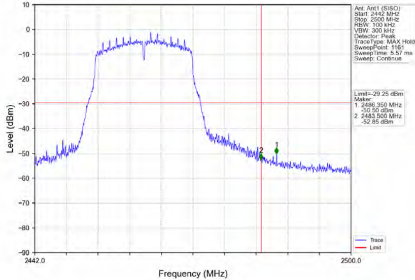
802.11n(HT20)_HCH_2462MHz_Ant1 (SISO)_NTNV
