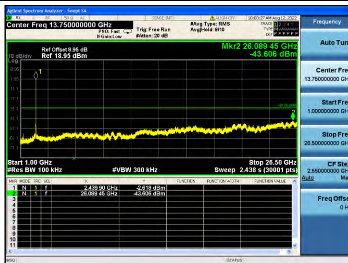
11N20MIMO_Ant1_2437_1000~26500
