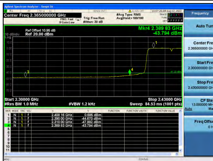
11N40MIMO_Ant1_Low_2422_AV
