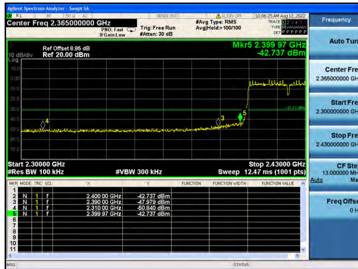
11N40MIMO_Ant2_Low_2422
