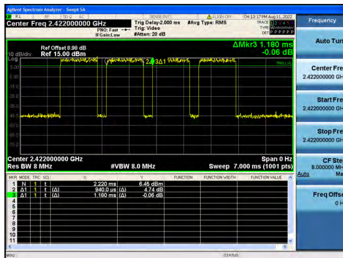
11N40MIMO_Ant2_2422
