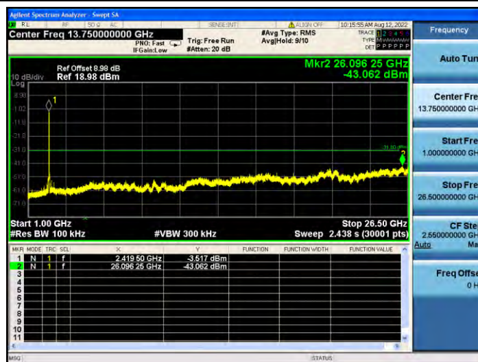
11N40MIMO_Ant2_2422_1000~26500
