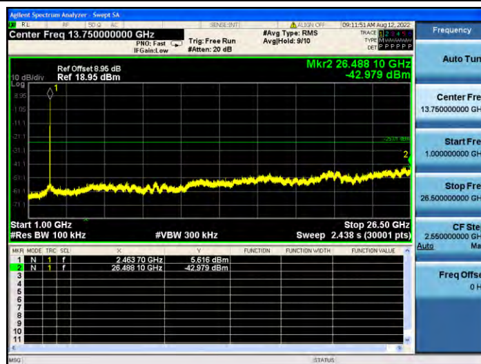
11B_Ant1_2462_1000~26500
