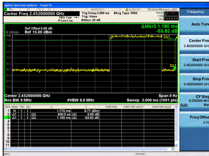
11N40MIMO_Ant2_2452
