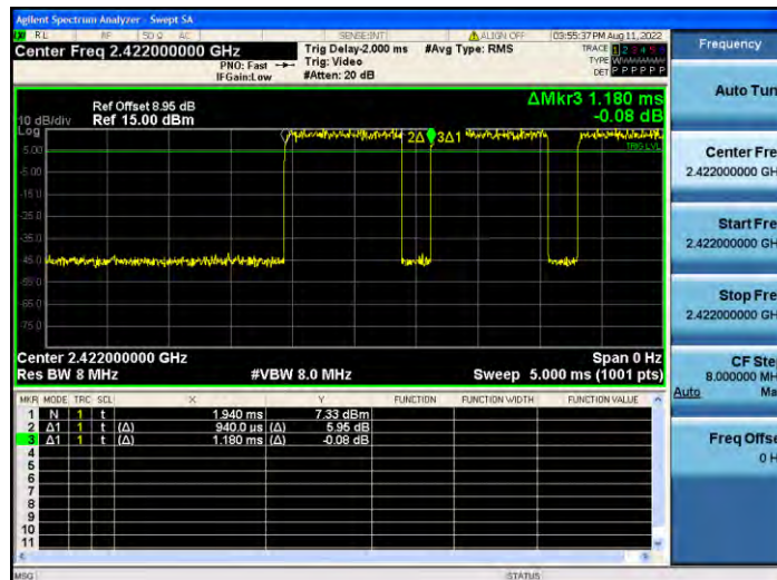
11N40MIMO_Ant2_2422
