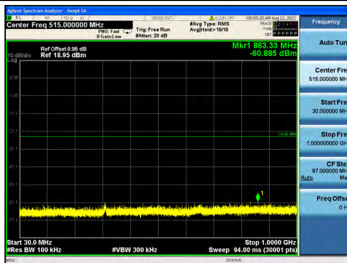
11B_Ant1_2437_30~1000
