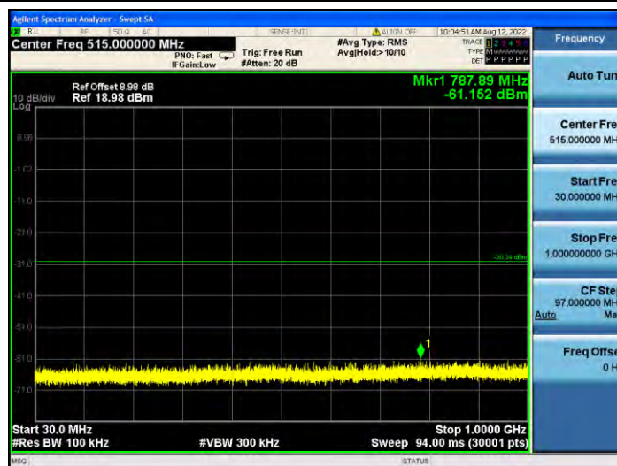
11N20MIMO_Ant2_2462_30~1000
