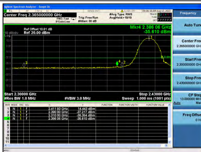
11B_Ant2_Low_2412_AV
