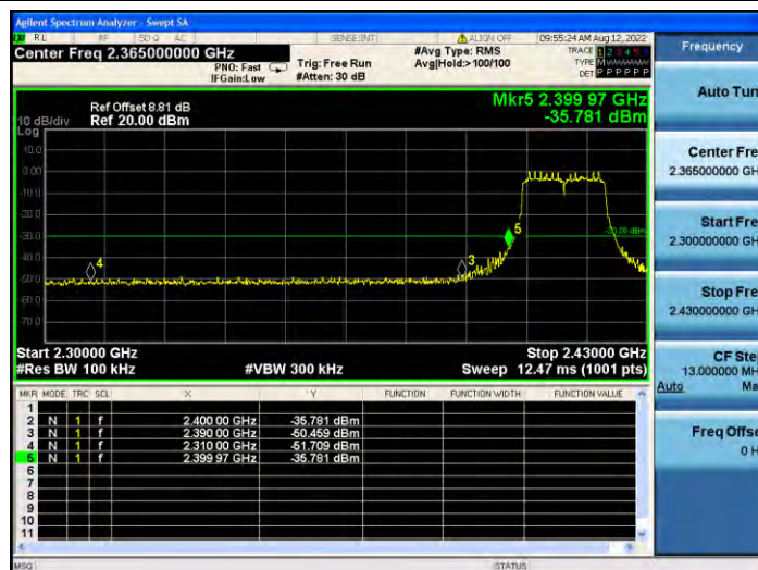
11N20MIMO_Ant2_Low_2412
