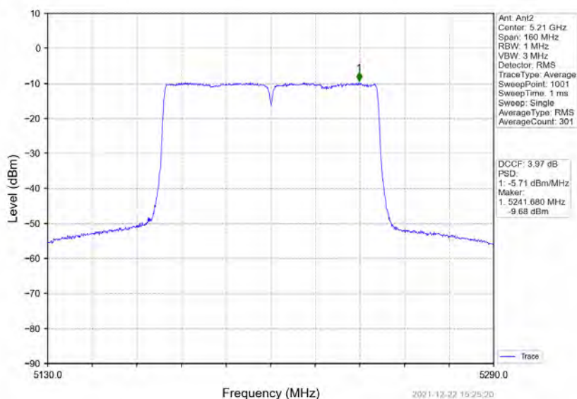
802.11ac(VHT80) MCH_5210MHz_MIMO_NTNV
