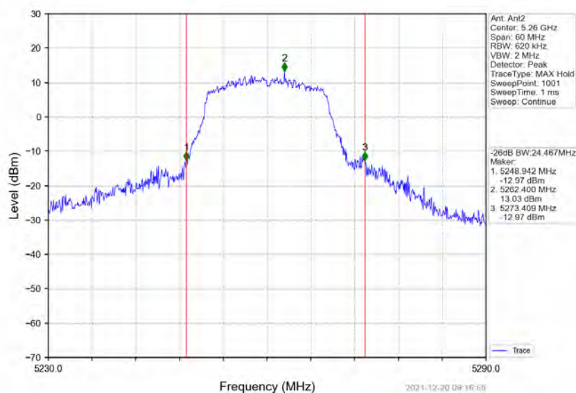
802.11a LCH_5260MHz_Ant2_NTNV
