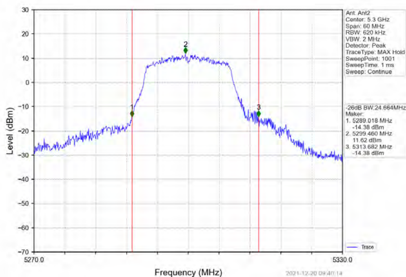
802.11a_MCH_5300MHz_Ant2_NTNV
