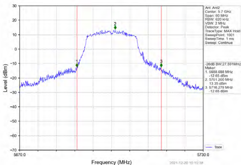
802.11a_HCH_5700MHz_Ant2_NTNV
