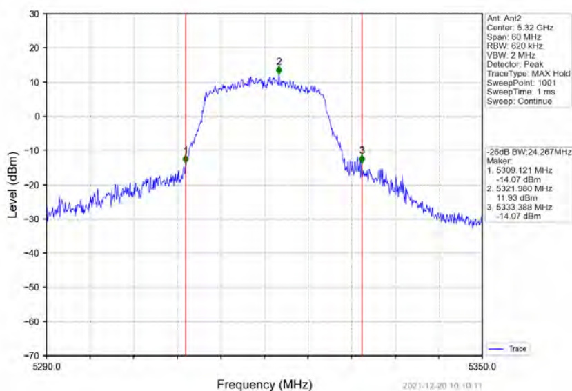
802.11a_HCH_5320MHz_Ant2_NTNV
