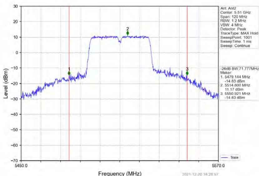
802.11ac(VHT40) LCH_5510MHz_Ant2_NTNV
