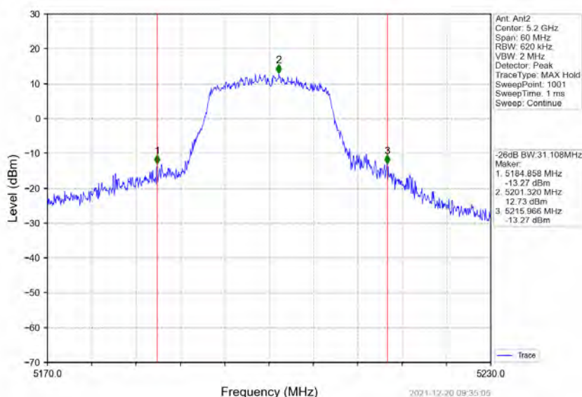
802.11a_MCH_5200MHz_Ant2_NTNV
