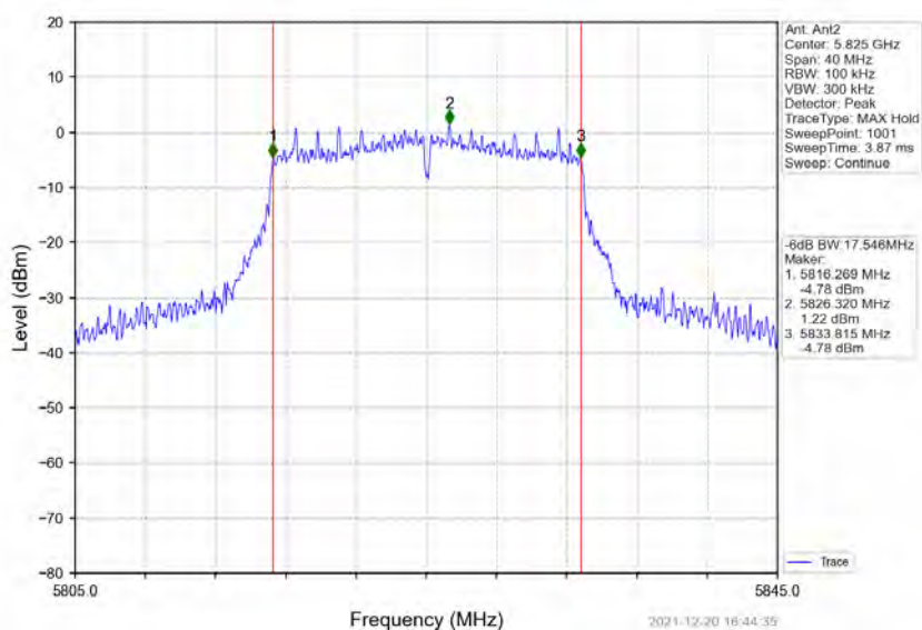
802.11ac(VHT20) HCH 5825MHz Ant2 NTV
