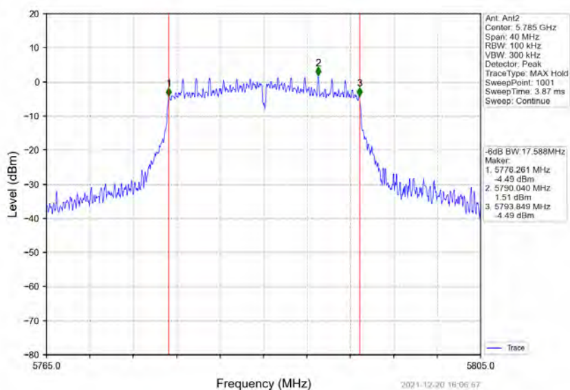
802.11ac(VHT20) MCH 5785MHz Ant2 NTV
