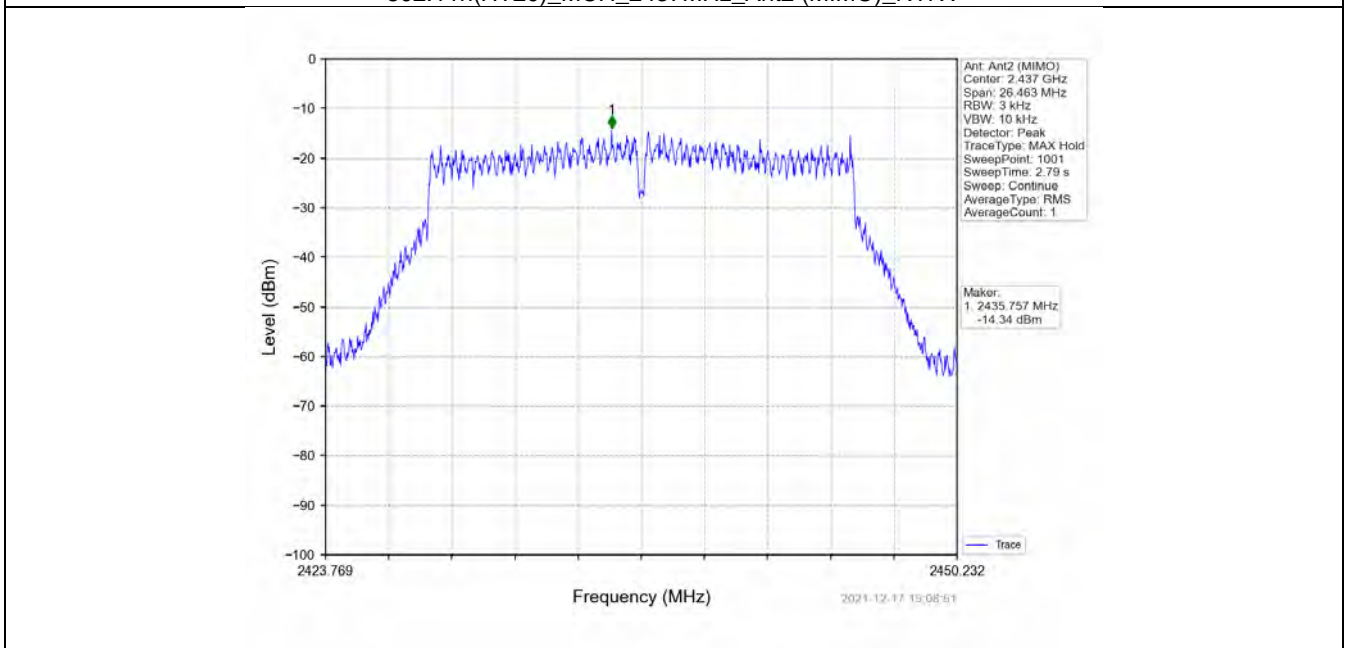
802.11n(HT20)_MCH_2437MHz_MIMO_NTNV
