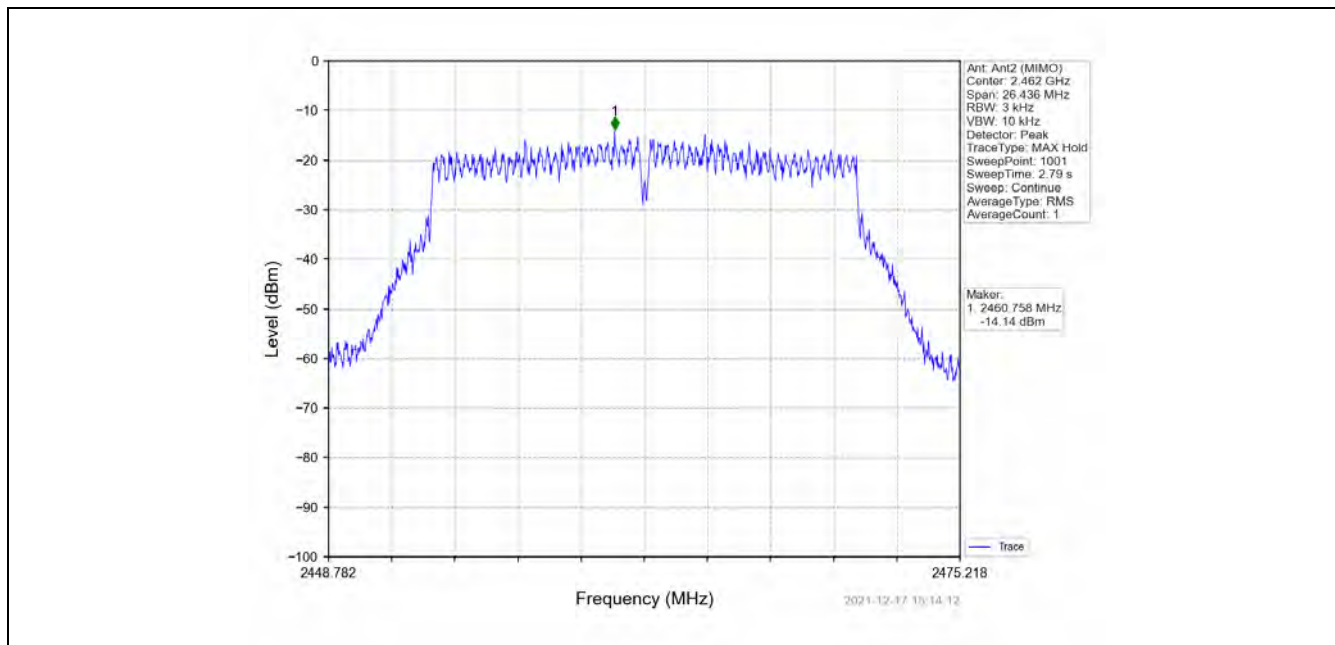
802.11n(HT20)_HCH_2462MHz_MIMO_NTNV
