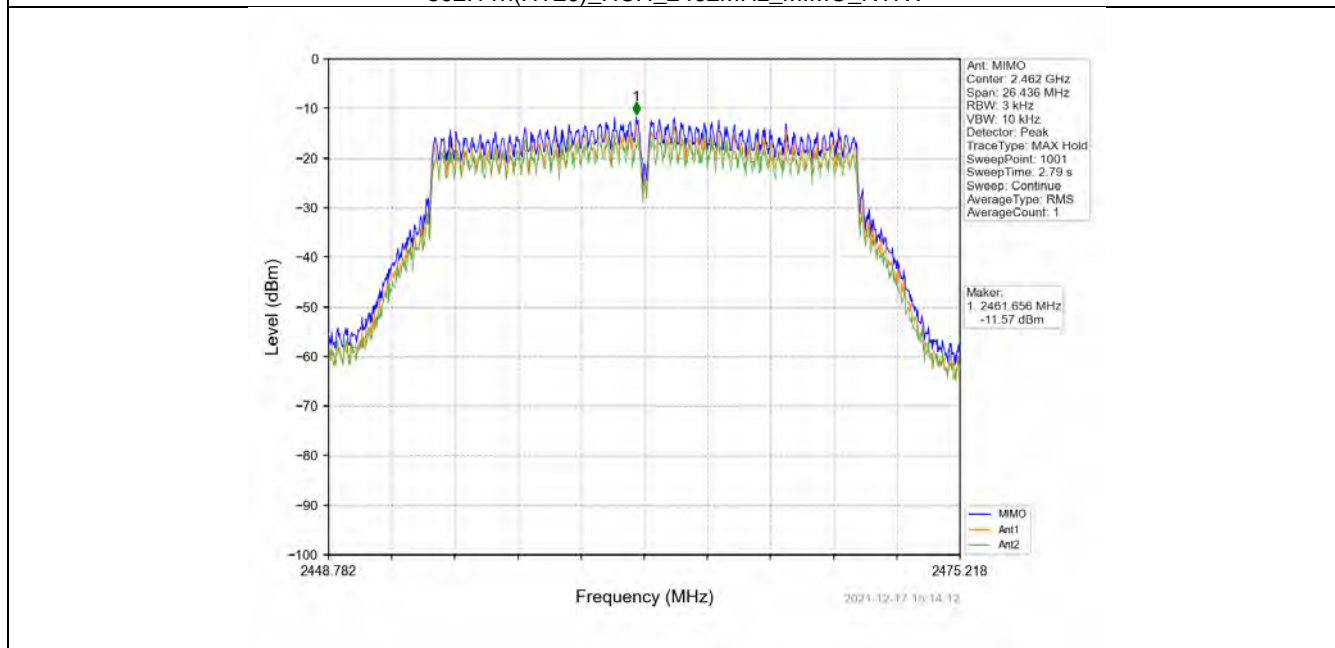
802.11n(HT20)_HCH_2462MHz_MIMO_NTNV
