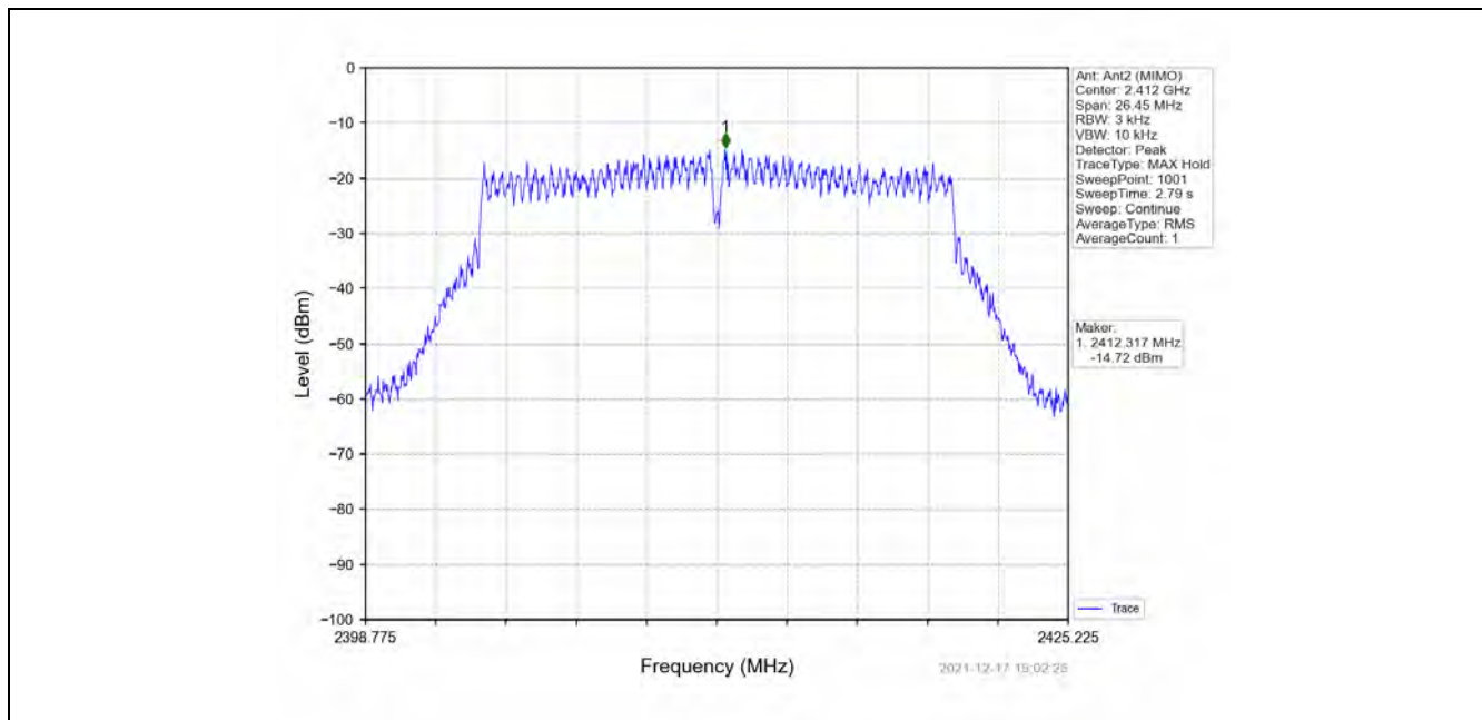
802.11n(HT20)_LCH_2412MHz_MIMO_NTNV
