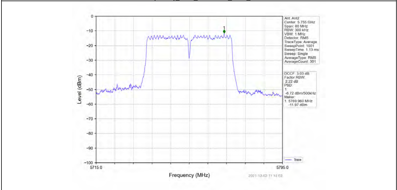
802.11n(HT40)_LCH_5755MHz_MIMO_NTNV
