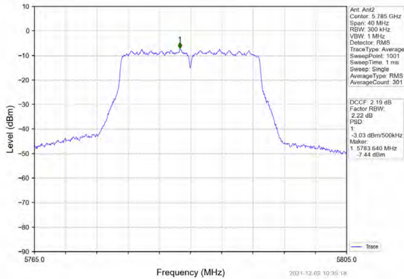
802.11n(HT20)_MCH_5785MHz_MIMO_NTNV
