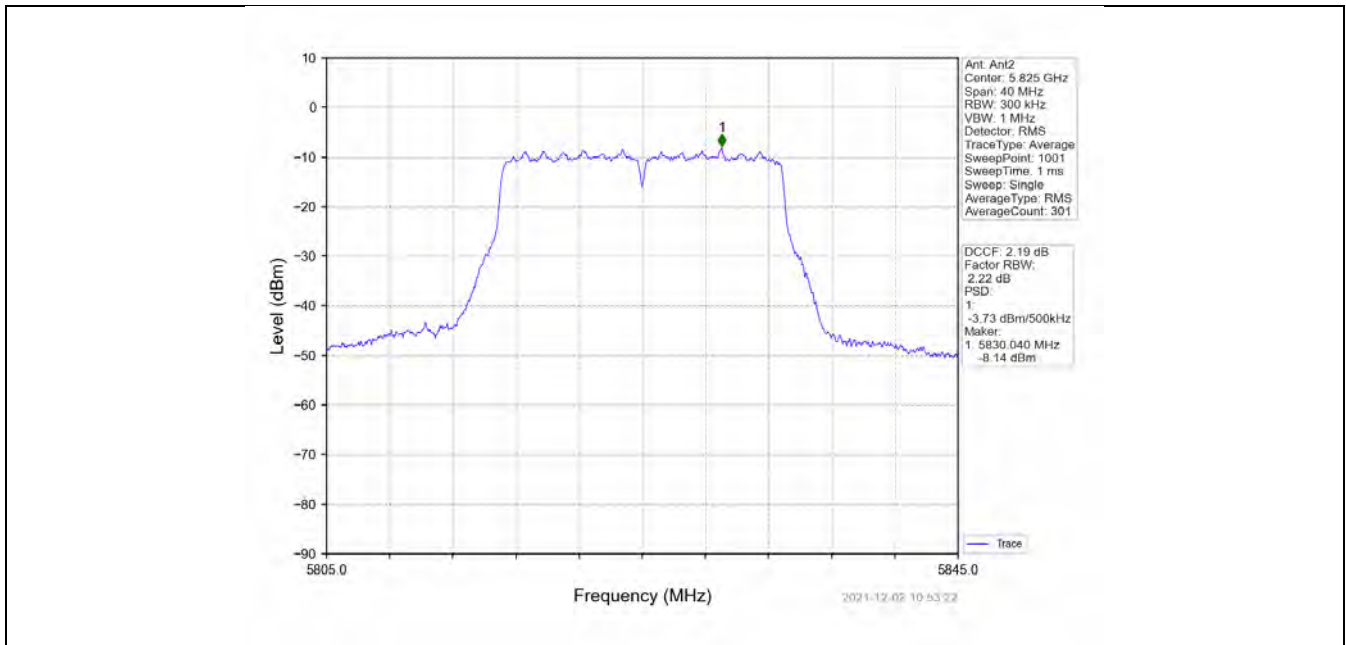
802.11n(HT20)_HCH_5825MHz_MIMO_NTNV
