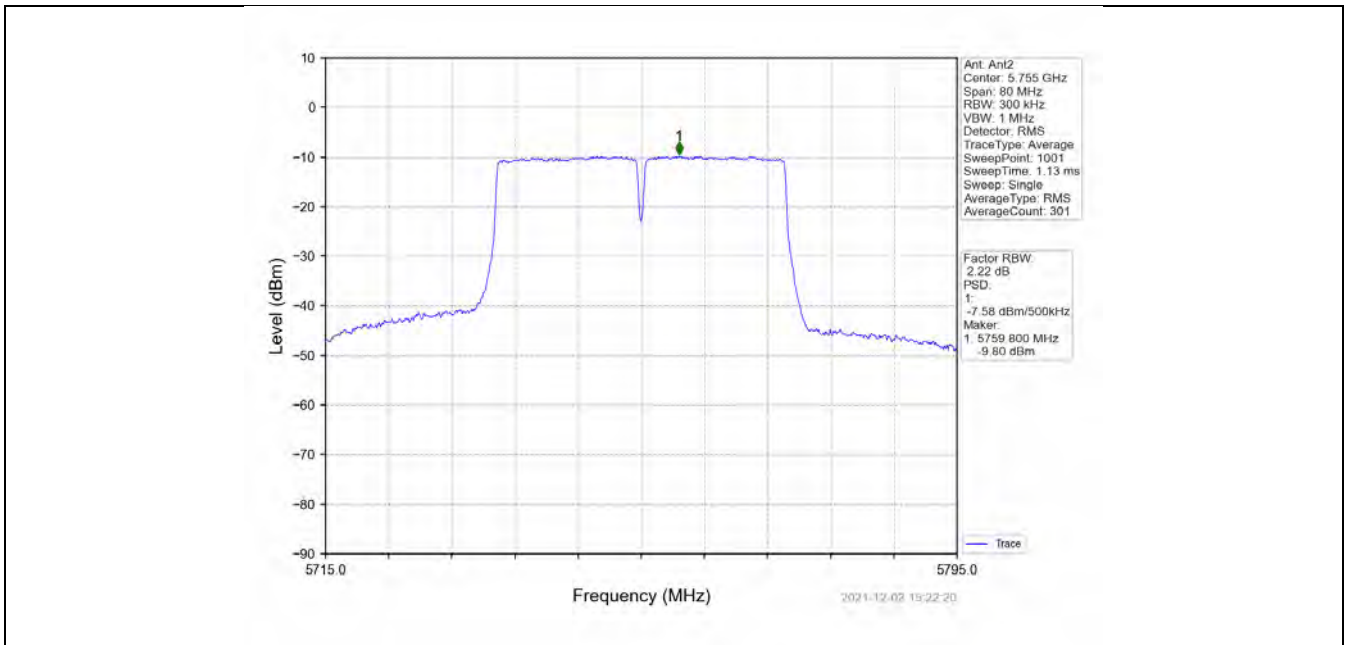
802.11ac(VHT40)_LCH_5755MHz_MIMO_NTNV
