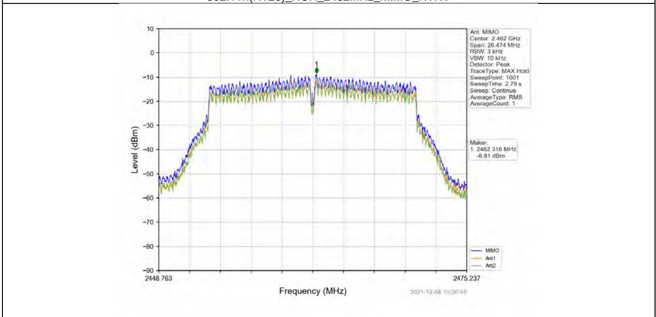
802.11n(HT20)_HCH_2462MHz_MIMO_NTNV
