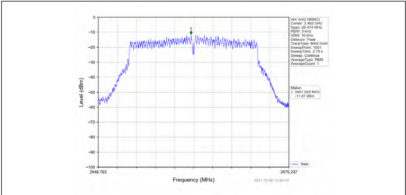
802.11n(HT20)_HCH_2462MHz_MIMO_NTNV
