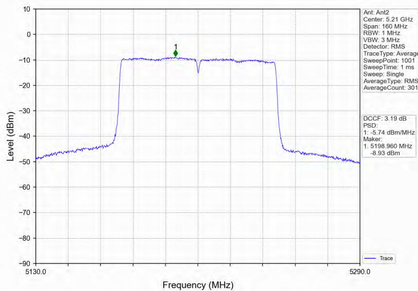
802.11ac(VHT80)_MCH_5210MHz_Ant2_NTNV
