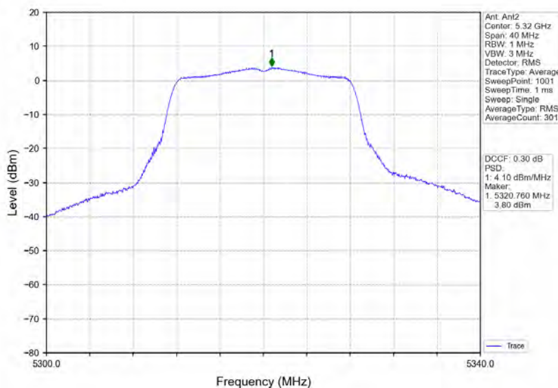
802.11a_HCH_5320MHz_Ant2_NTNV
