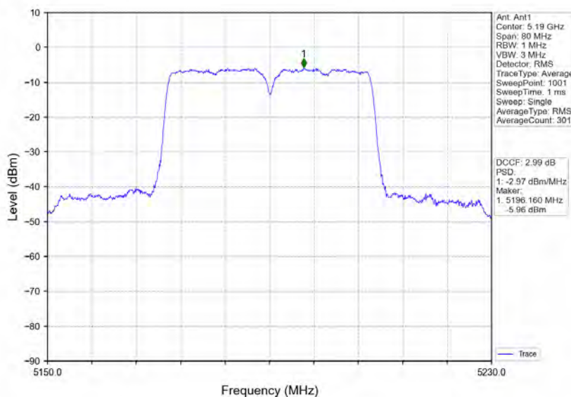
802.11n(HT40)_LCH_5190MHz_Ant1_NTNV
