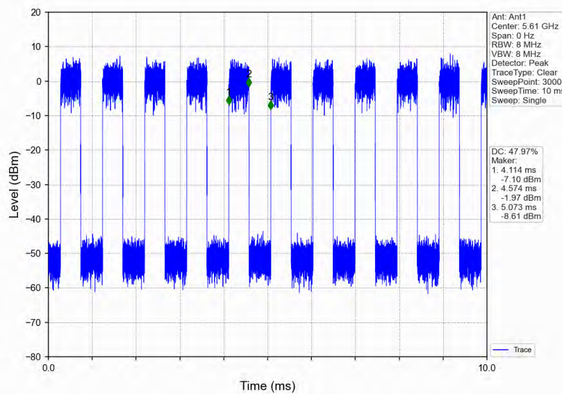
802.11ac(VHT80)_HCH_5610MHz_Ant1_NTNV
