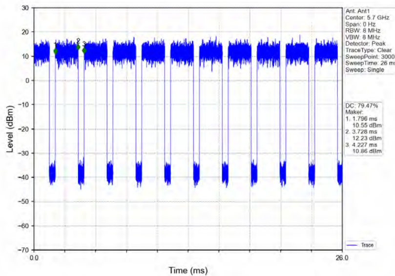
802.11ac(VHT20)_HCH_5700MHz_Ant1_NTNV
