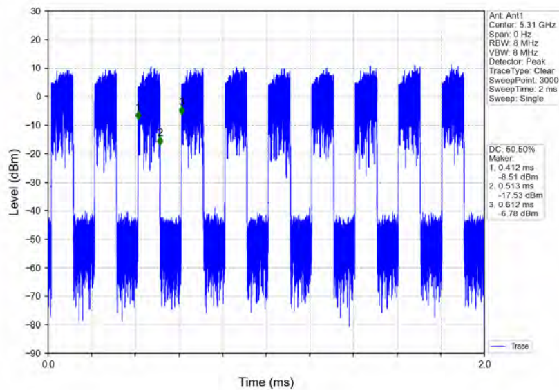
802.11n(HT40)_HCH_5310MHz_Ant1_NTNV
