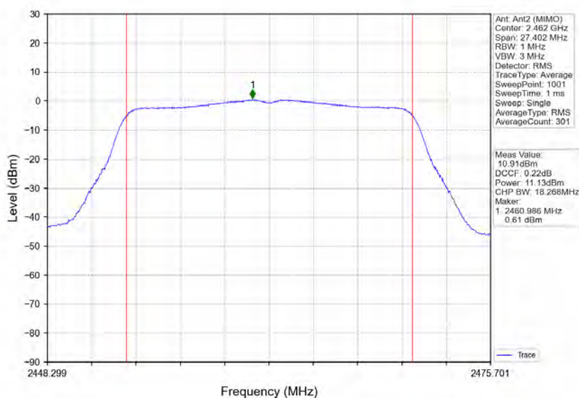
802.11n(HT20)_HCH_2462MHz_Ant2 (MIMO)_NTNV
