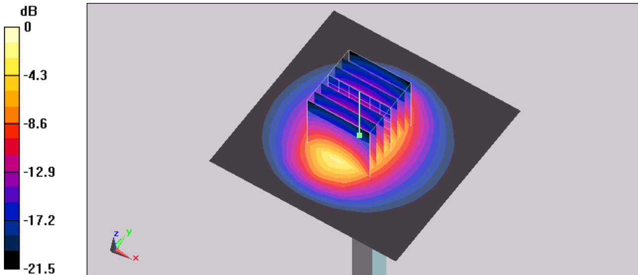
0 dB = 5.76mW/g
