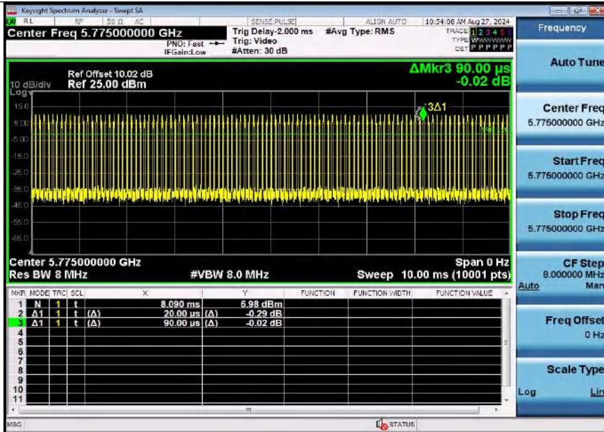
NTNV-11AC80SISO-Ant1-5775
