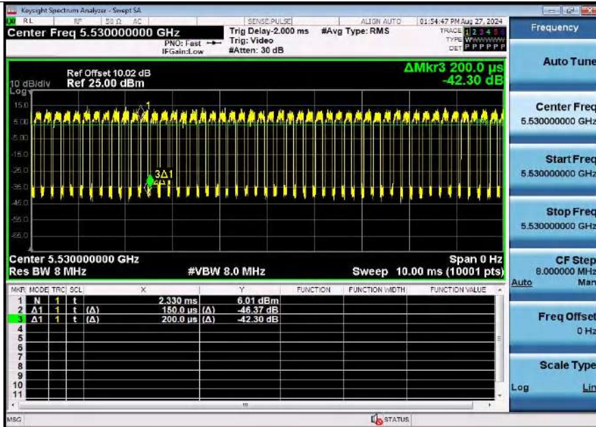
NTNV-11AX80SISO-Ant1-5530
