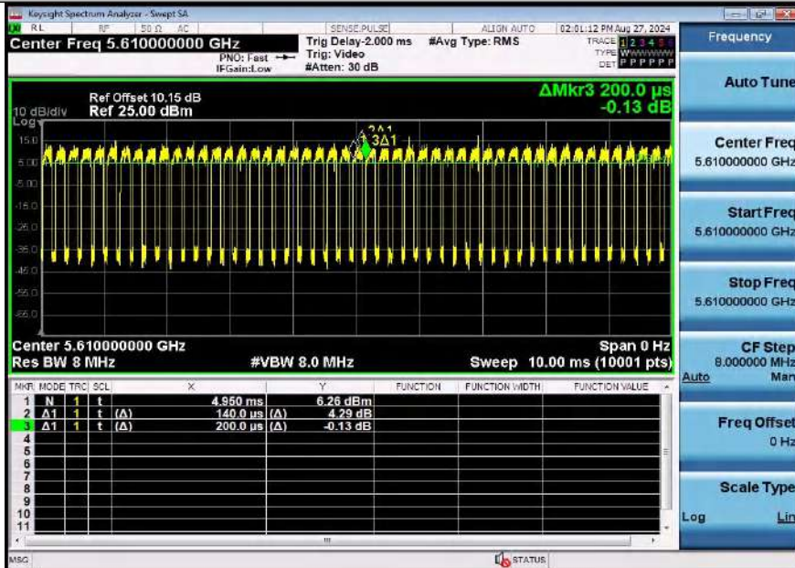
NTNV-11AX80SISO-Ant1-5610
