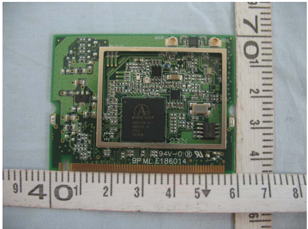
(4) EUT Photo
