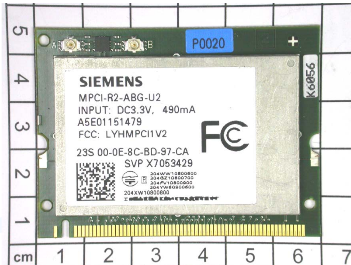
WLAN module
