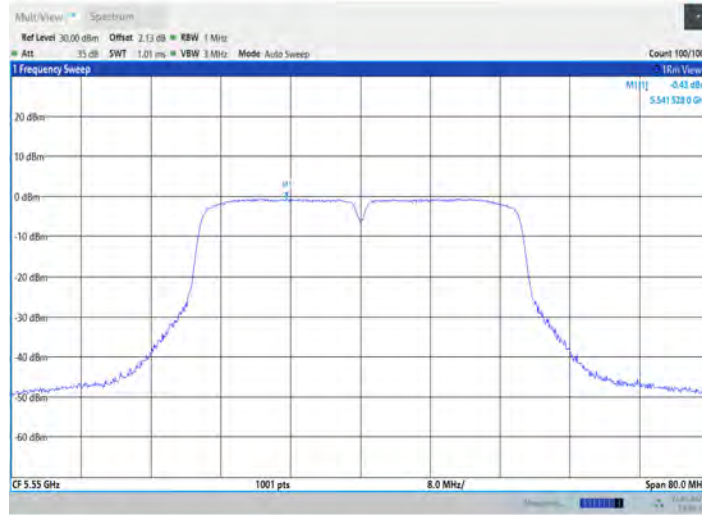
11n40SISO_Ant1_5550
