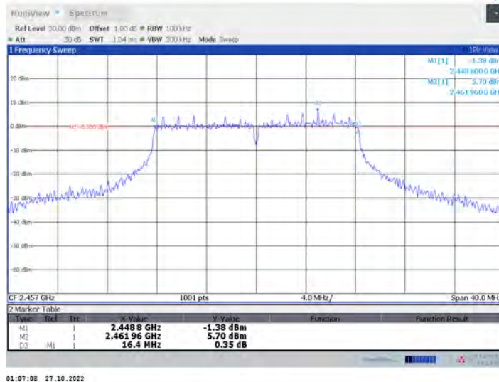
11g_Ant1_2457
