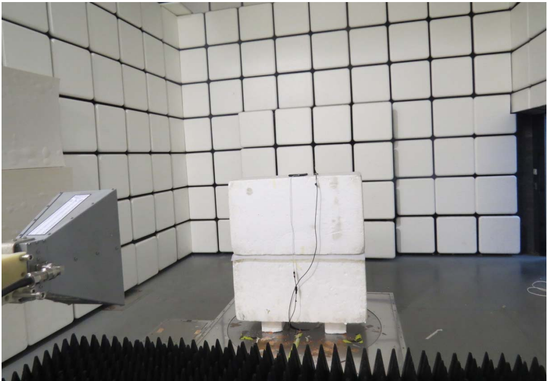
1GHz-18GHz
