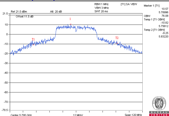
802.11n (HT40)_Chain1 / CH159
