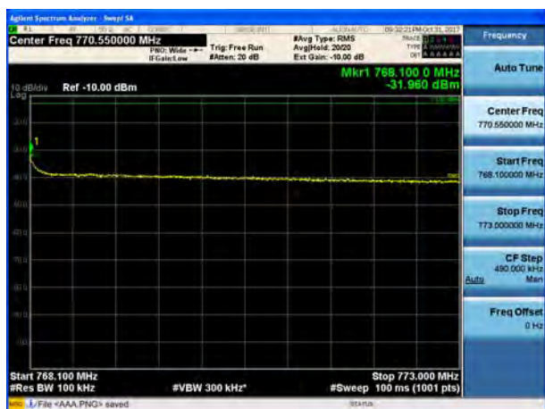
768.1 MHz ~ 773 MHz
