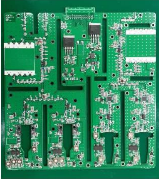
Top Layer
