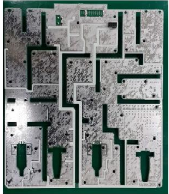
Bottom Layer
