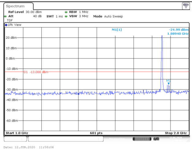
1GHz-2GHz
