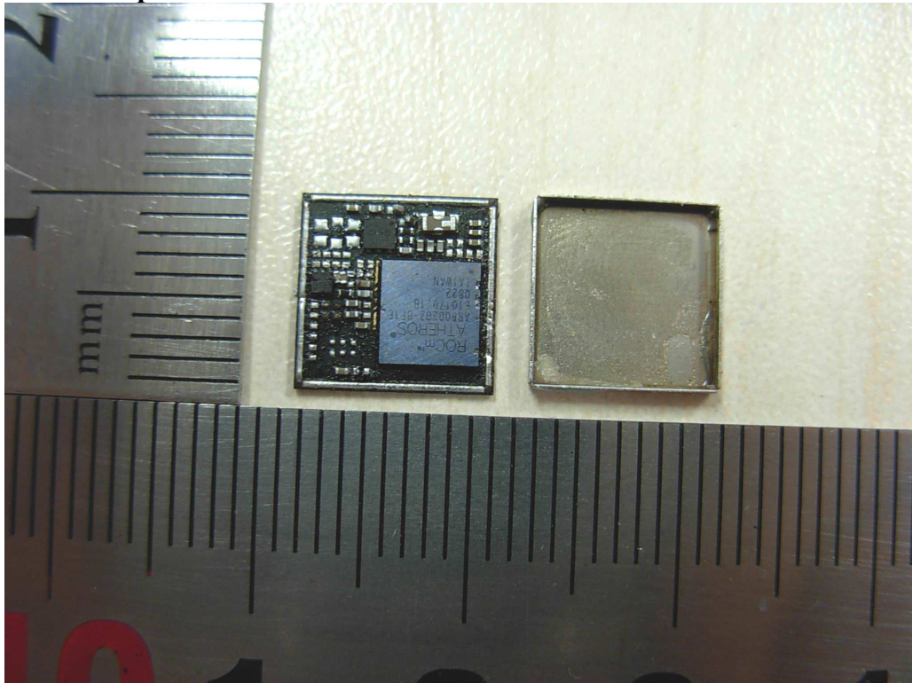
Wi-fi IC top view
