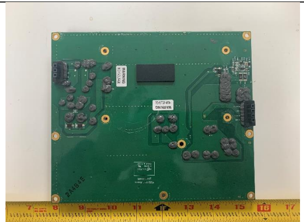
EUT-PCBA2-Bottom
