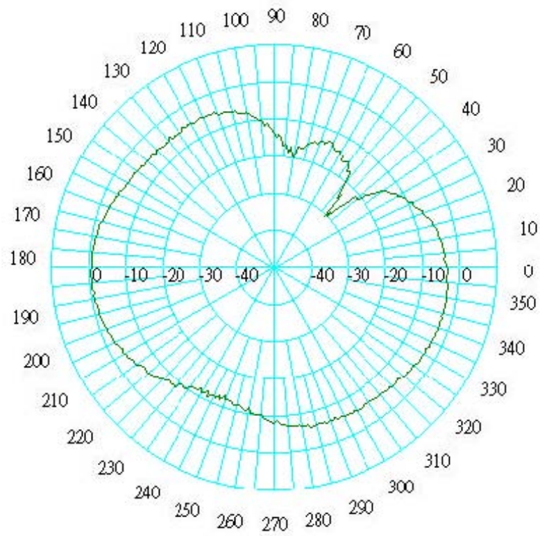
2.45-H.ant 2.48-E.ant
