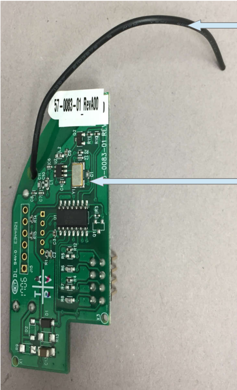
Antenna
