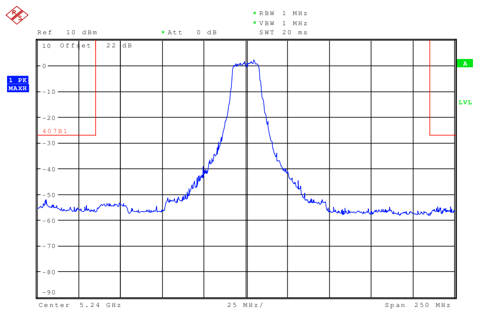
Plot 2: upper band edge
