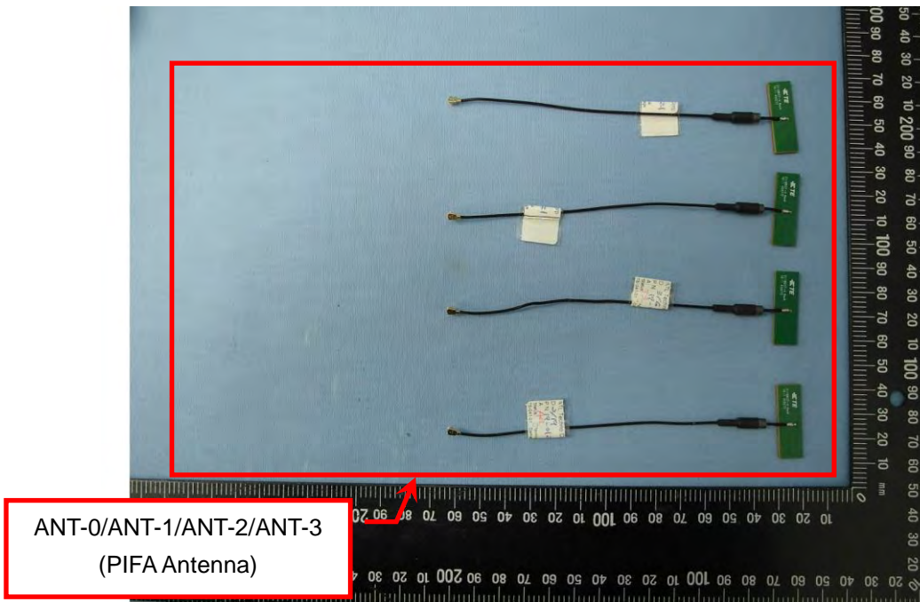
EUT Photo (2)
